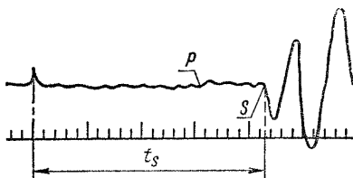
S—начало первой фазы колебаний поперечных волн
