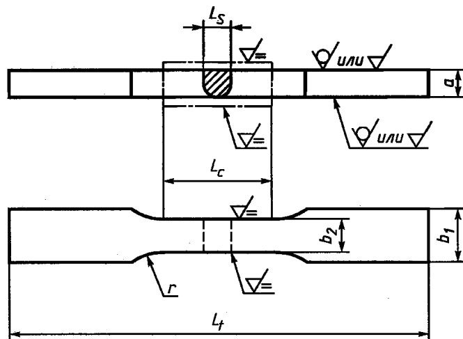
Черт. 2. Образец для испытаний
