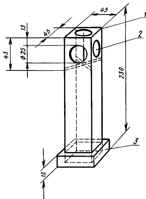
Прибор для измерения концентрации пыли
