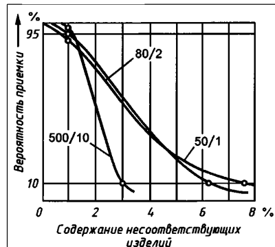
Кривые оперативных характеристик для планов выборочного контроля
