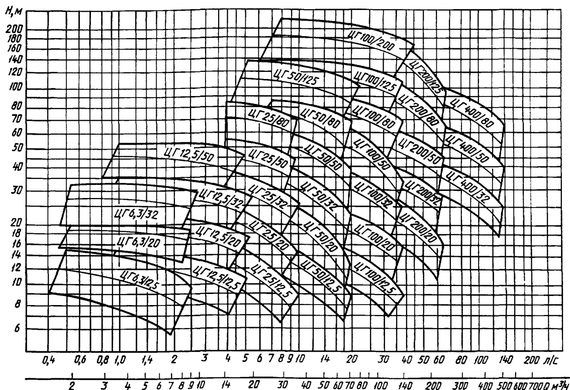
Поля Q-H
