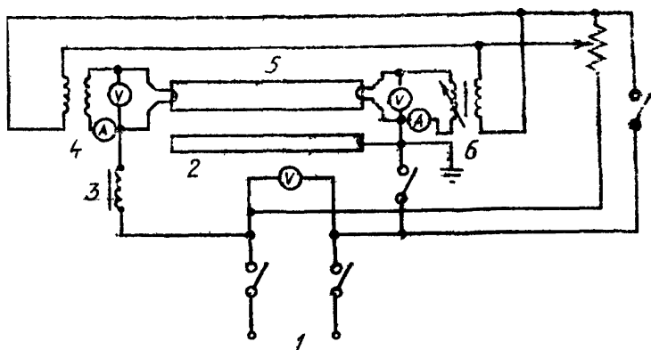
1 — источник питания; 2 — зажигающая полоса; 3 — балласт; 4, 6 — трансформаторы; 5 — лампа
