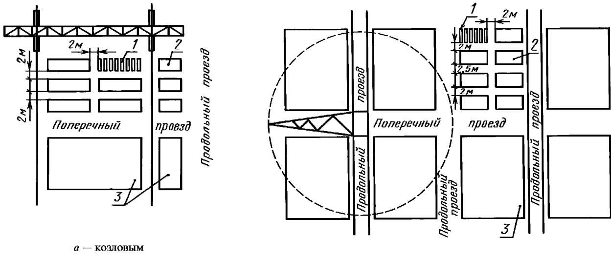
б — башенным
