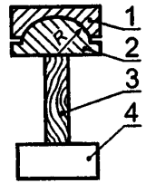
1, 2 — самоустанавливающиеся пластины; 3 — образец; 4 — нижняя платформа испытательной машины
