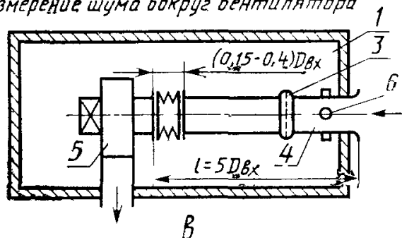
Измерение шума вокруг вентилятора
