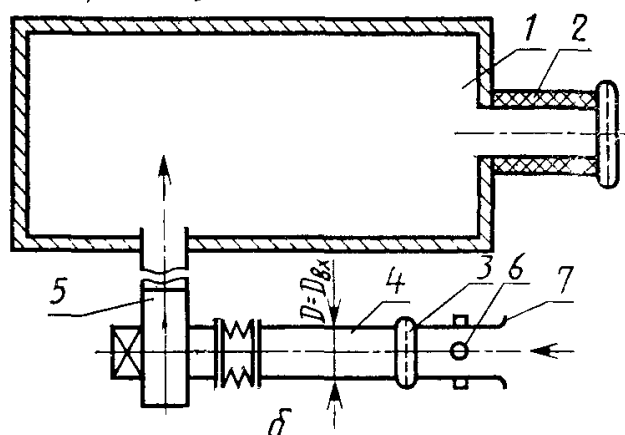
Измерение шума вокруг вентилятора
