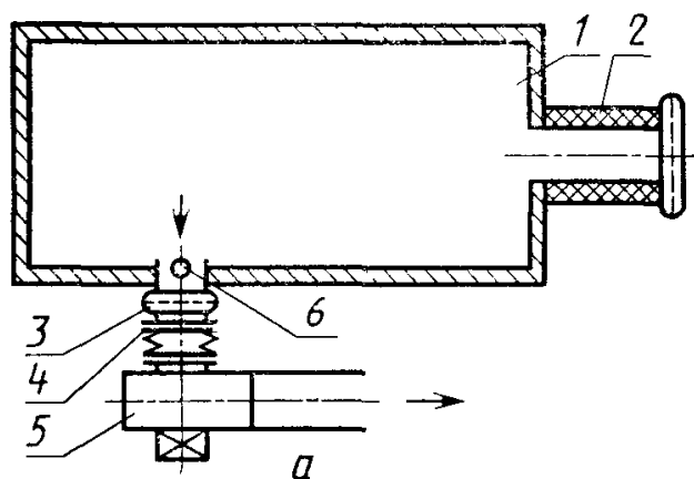
Измерение шума нагнетания
