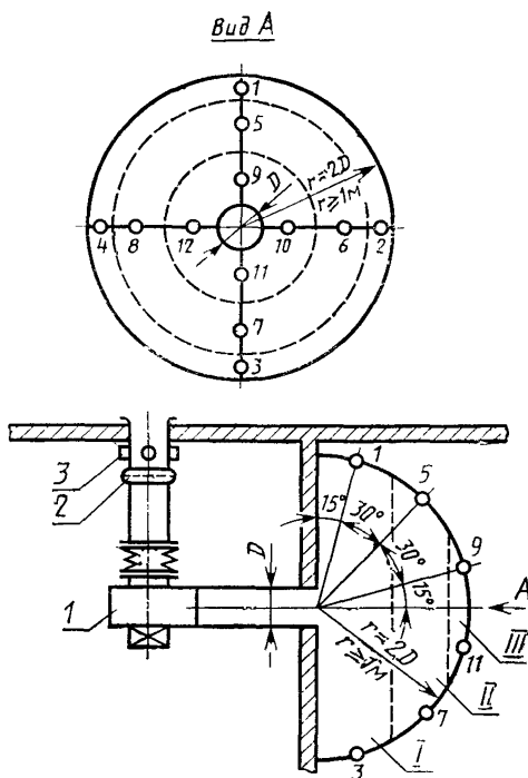
1 — испытуемый вентилятор; 2 — дросселирующее устройство; 3 — место измерения производительности; I, II, III — измерительные пояса; о — измерительная точка
