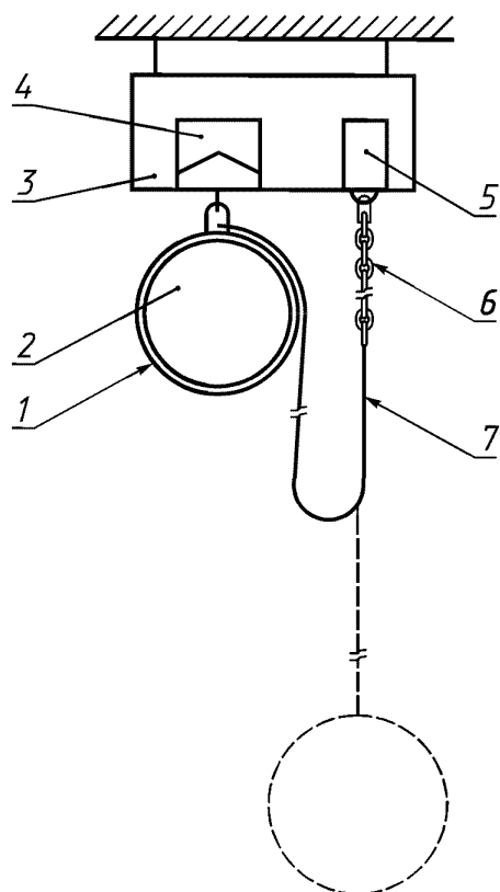
1 — пояс; 2 — груз или манекен массой 100 кг; 3 — подъемное устройство; 4 — распепляющее устройство; 5 — датчик измерительного устройства; 6 — технологический фал для удлинения стропы до 2 м или до двух длин стропы; 7 — стропы
