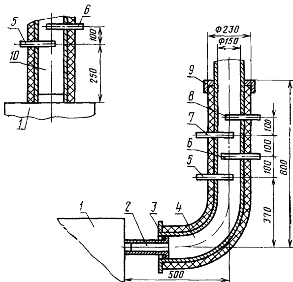
1—аппарат, 2—переходник, 3—шнур асбестовый, 4—труба для горизонтального подсоединения, 5—пробоотборник, 6—термометр, 7—трубка для измерения разрежения, 8—трубка для отбора сажистых частиц, 9—крышка, 10—труба для вертикального подсоединения
