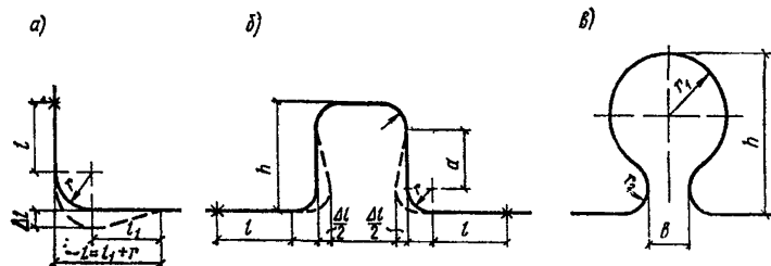
Рис. 3. Основные геометрические параметры а — гнutoго отвода; б — П-образного компенсатора; в — лирообразного компенсатора
