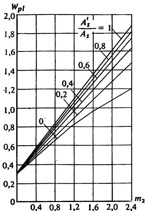
Черт. 3. График значений коэффициента W_{pl} для определения момента появления трещин M_{pl} в изгибаемых элементах прямоугольного сечения при \delta = 0,1
