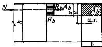
Черт. 1. Схема усилий и эпюра напряжений в сечении, нормальном к продольной оси внецентренно сжатого бетонного элемента, рассчитываемого по прочности без учета сопротивления бетона растянутой зоны
