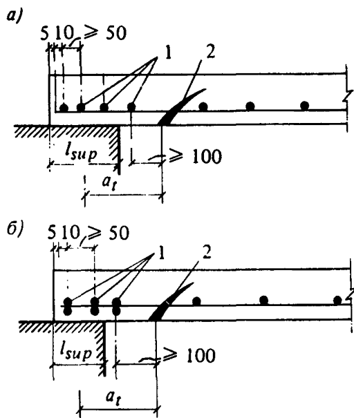
Черт. 11. Примеры анкеровки арматуры плит из ячеистого бетона на опорах растянутых стержней
