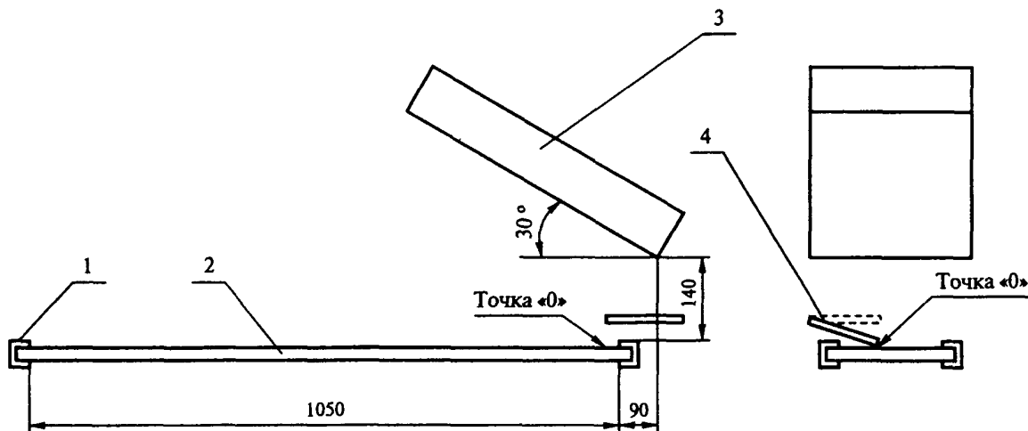
1 — держатель; 2 — образец; 3 — радиационная панель; 4 — газовая горелка
