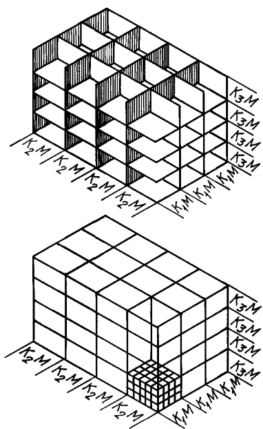
Прямоугольная модульная пространственная координационная система
