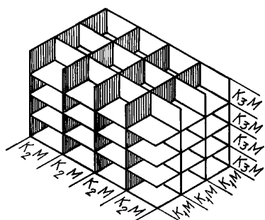
Прямоугольная модульная пространственная координационная система
