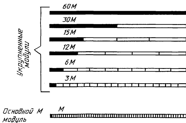
Взаимосвязь между модулями различной крупности
