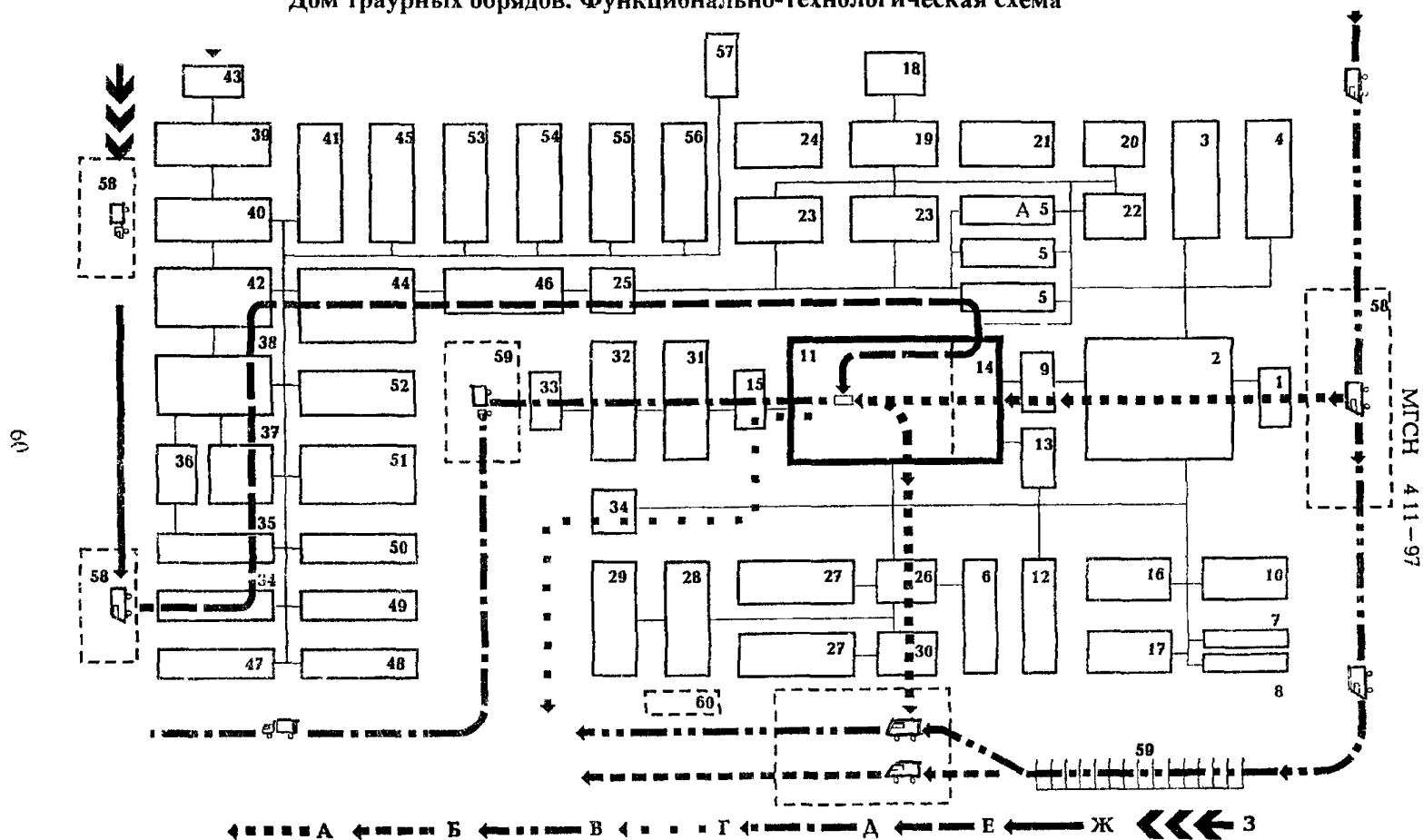
Дом траурных обрядов. Функционально-технологическая схема
