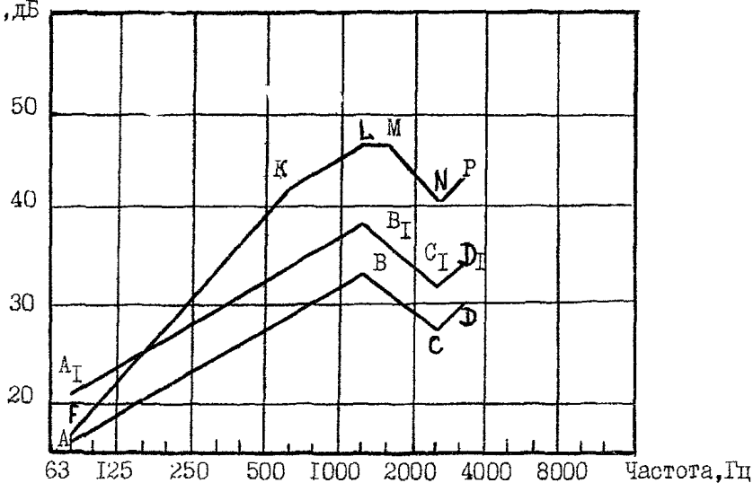
Рис. 3.8. Расчетная частотная характеристика к примеру 8
