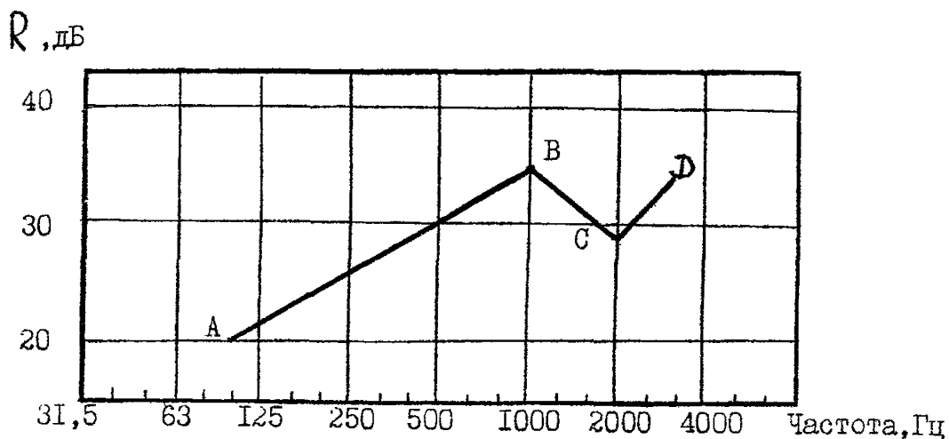
Рис. 3.5. Расчетная частотная характеристика к примеру 7.
