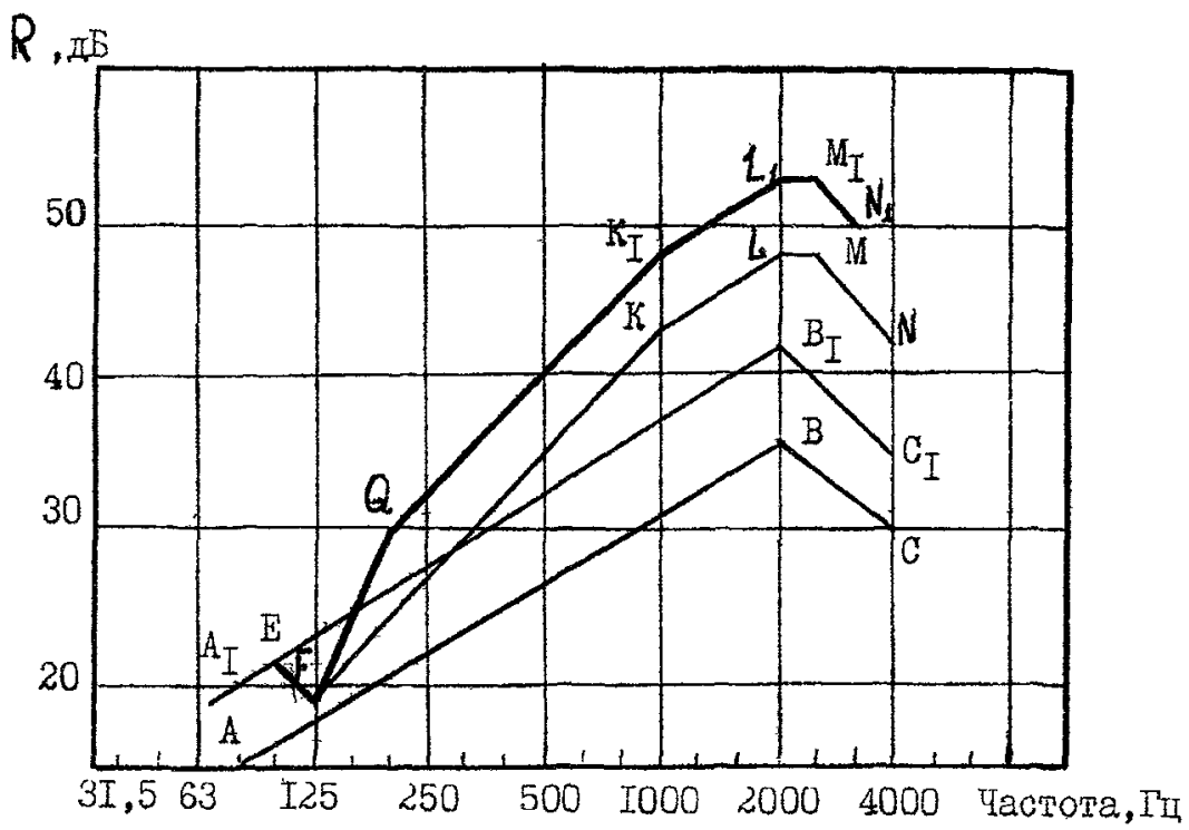
Рис. 3.11. Расчетная частотная характеристика к примеру 10
