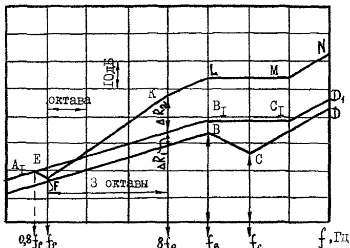
Рис. 3.7. Частотная характеристика изоляции воздушного шума конструкции, состоящей из двух листов с воздушным промежутком между ними при различной толщине листов
