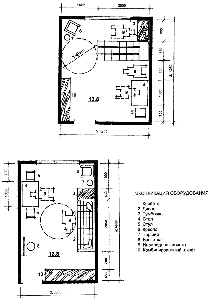
РИС.4.1. ПЛАНИРОВОЧНЫЕ СХЕМЫ ОДНОМЕСТНОЙ СПАЛЬНОЙ КОМНАТЫ
