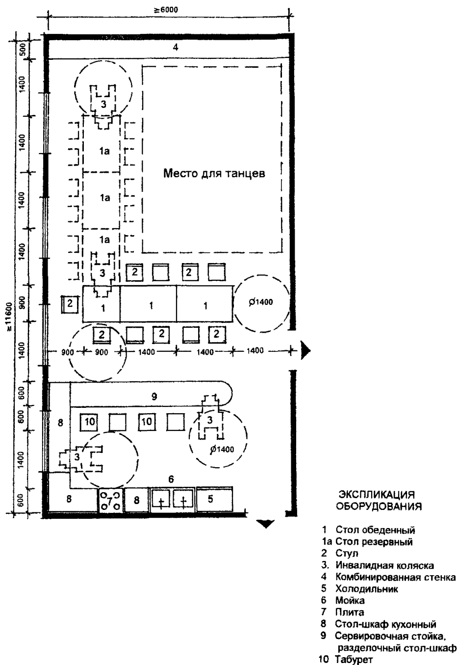
РИС 5 1 ПЛАНИРОВОЧНАЯ СХЕМА КАБИНЕТА СОЦИАЛЬНО-БЫТОВОЙ АДАПТАЦИИ, КОМНАТА ДЛЯ ПРИЕМА ГОСТЕЙ НА 11 И 21 ПОСАДОЧНЫХ МЕСТА
