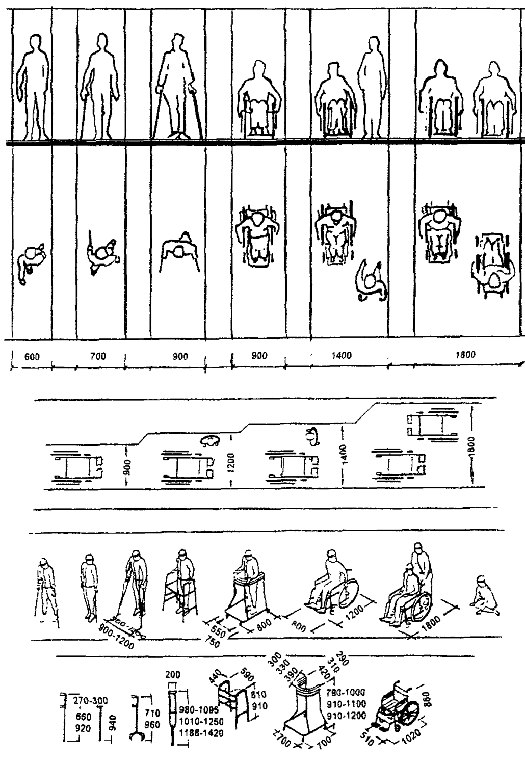
РИС.3.4 НЕОБХОДИМЫЕ ГАБАРИТЫ КОММУНИКАЦИЙ, УСТРОЙСТВ И СРЕДСТВ ПЕРЕДВИЖЕНИЯ ИНВАЛИДОВ
