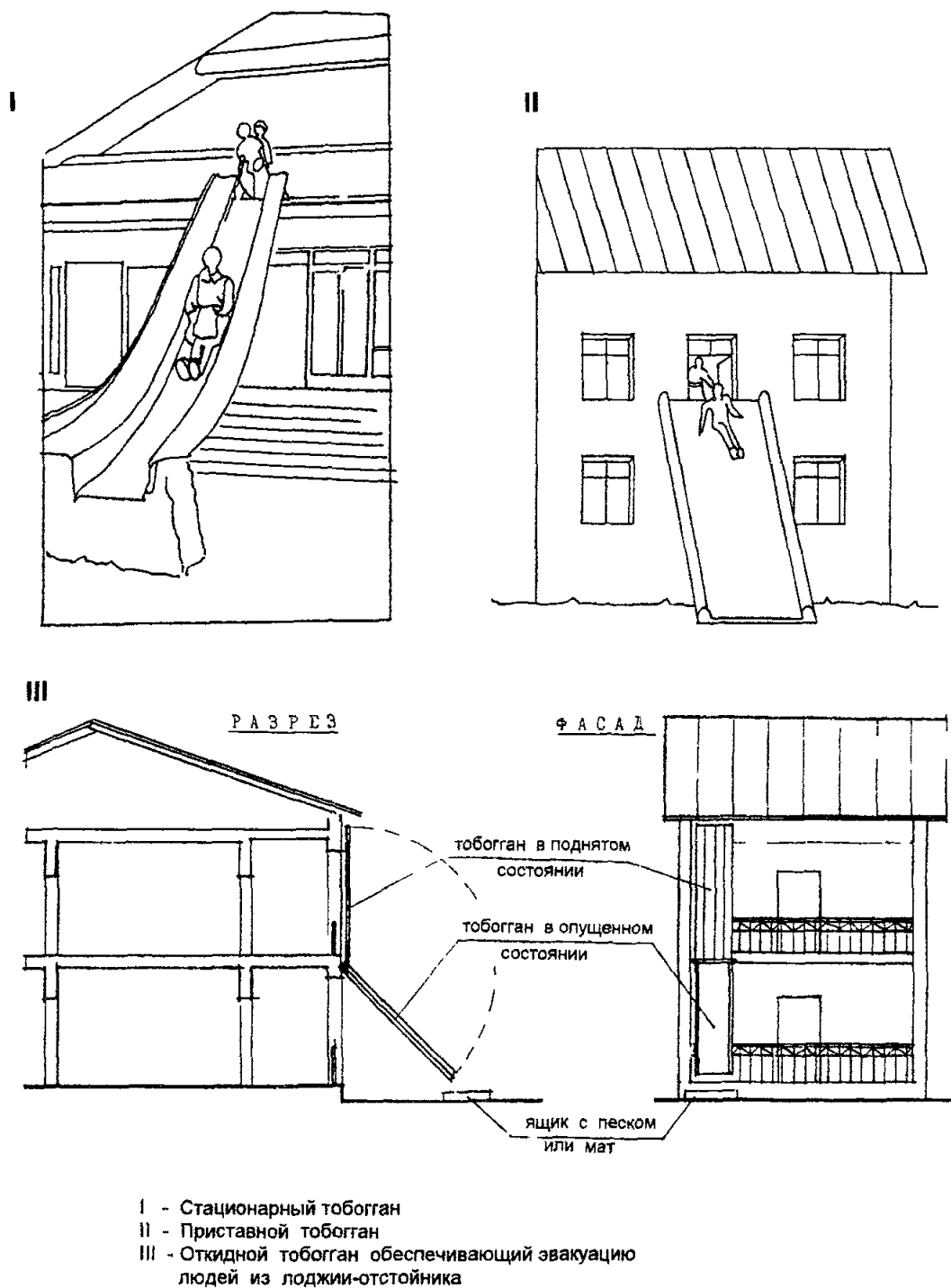
РИС 3 9 ТИПЫ ТОБОГГАНОВ ИСПОЛЬЗУЕМЫХ ДЛЯ ЭВАКУАЦИИ НА СЛУЧАЙ ПОЖАРА
