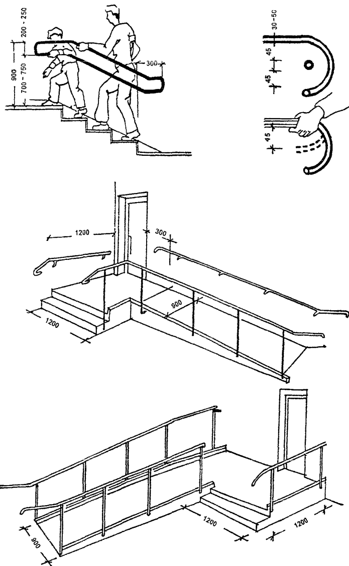
РИС. 3.11. ПРИМЕРЫ УСТРОЙСТВА ВХОДНЫХ ЛЕСТНИЦ И ПАНДУСОВ, РАСЧИТАННЫХ НА ИНВАЛИДОВ
