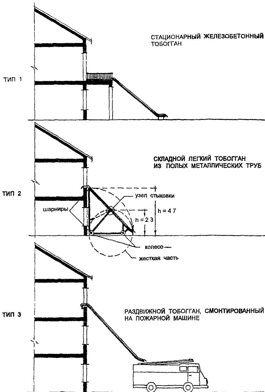
РИС. 3.13 СХЕМЫ ТОБОГАНОВ
