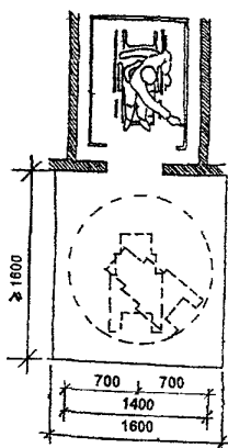
РИС.3 7 ГАБАРИТНЫЕ СХЕМЫ ПАНДУСОВ, ПОВОРОТОВ В КОРИДОРАХ, ОТКРЫВАНИЯ ДВЕРЕЙ, ЛИФТОВЫХ ПЛОЩАДОК, ЛИФТОВЫХ ДВЕРЕЙ
