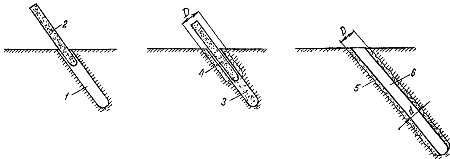
Рис.2.2. Схема изготовления щебеночной свай.
