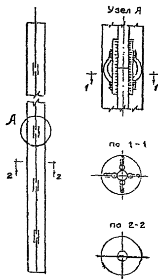
Рис. 8.2. Возможный вариант армирования буройнъекционных свай, воспринимающих нагрузку до 200 кН
