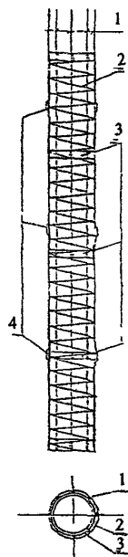
Рис. 8.1. Объемный арматурный каркас буронабивных, буросекущих и буронагнетационных свай
