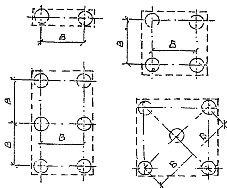
Рис. 8.3. Кустовое размещение бурабазивных свай B \geq 3D при D \leq 0,5 м B \geq 1 \text{ м} + D при D > 0,5 м
