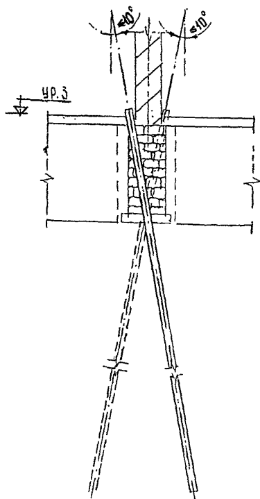
Рис. 8.4. Козловые фундаменты из буроналивных свай
