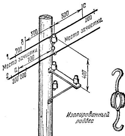
9.21. Устройство скрещивания на действующих цепях при помощи Г-образного кронштейна (1-я операция)
