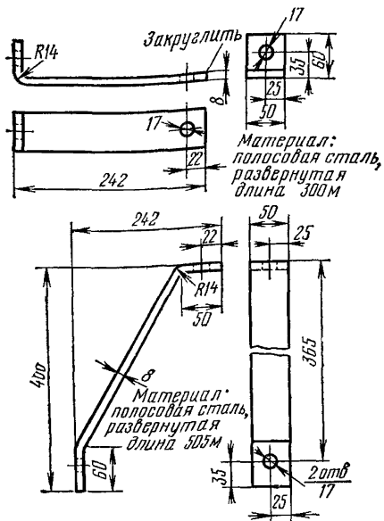
8 24. Траверса для кронштейна, применяемого на линиях РС или СТС
