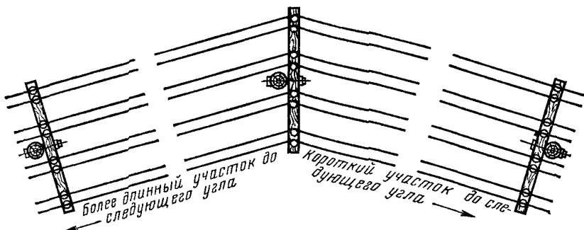
6.40. Расположение траверс на угловых и смежных с ними опорах
