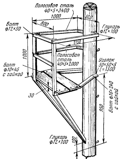
4.49. Кабельная площадка для одинарной и ш двуслойной опоры
