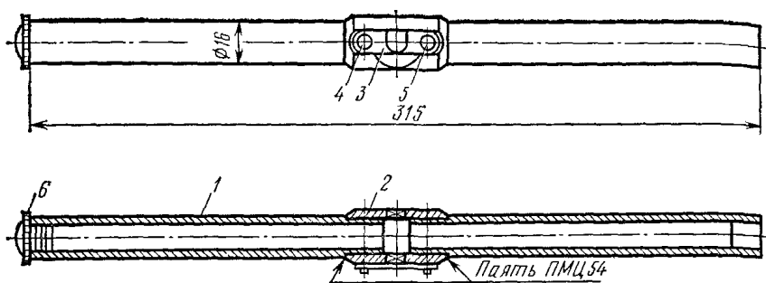
Рис. П.4.3. Ручка-футляр в сборе:
