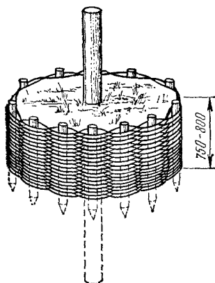
4.56. Устройство ряжа из местных материалов
