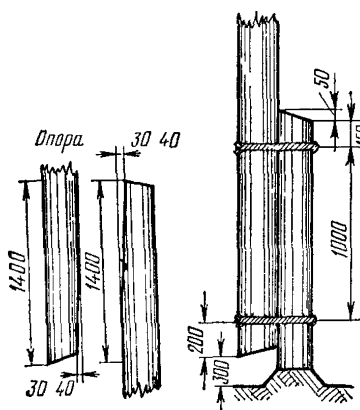
4.62. Укрепление опор одной деревянной приставкой
