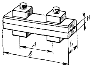
2.29. Двухболтовый зажим
