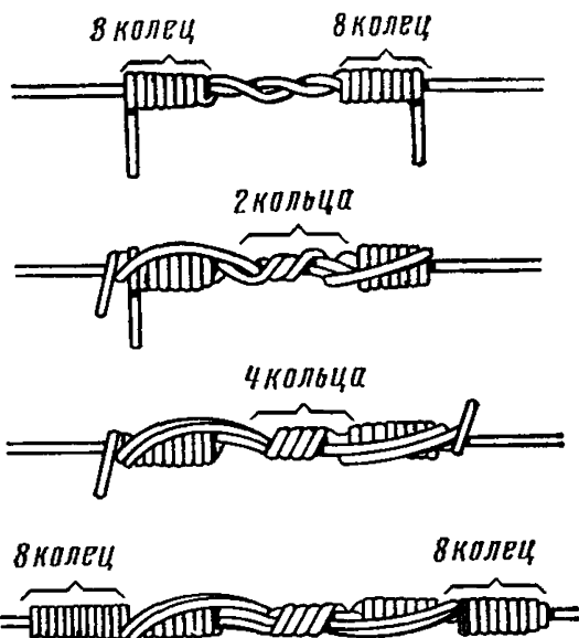
6.55. Скрутка проводов
