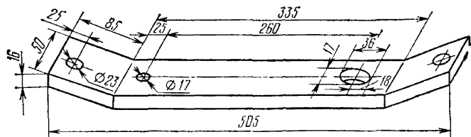
2.16. Двусторонняя накладка для особо усиленной конструкции крепления проводов
