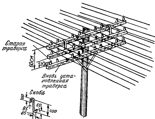
9.16. Замена верхней траверсы
