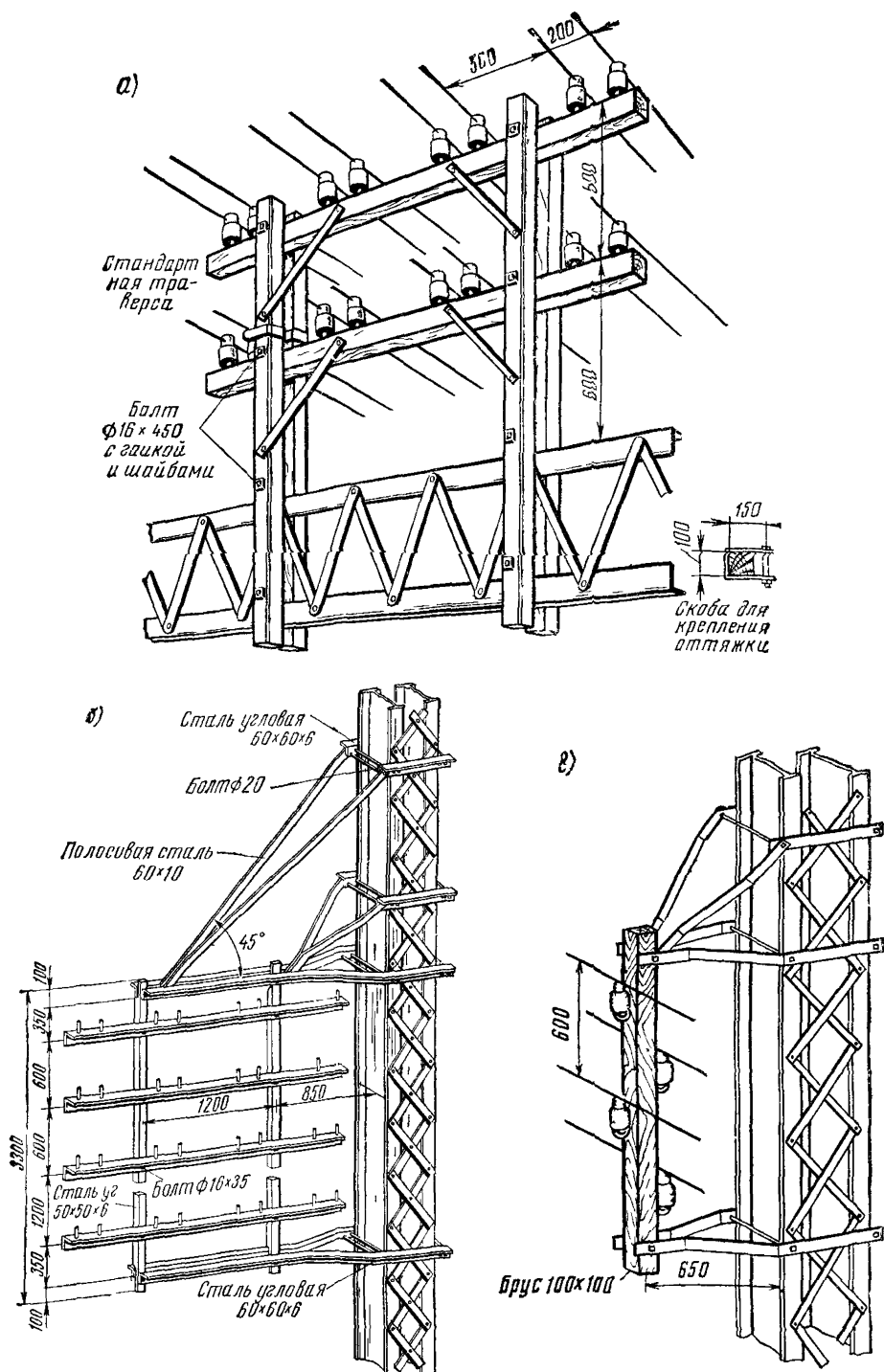
7.13. Конструкции мостового кронштейна для мостов
