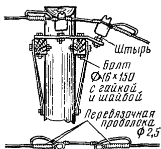
6.4. Особо усиленная конструкция крепления провода при одностороннем тяжении вниз
