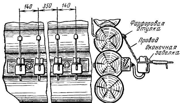
8.26. Устройство ввода при числе проводов не более восьми
