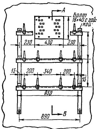
8.23. Устройство ввода на линиях РС или СТС (для небольшого количества проводов)
