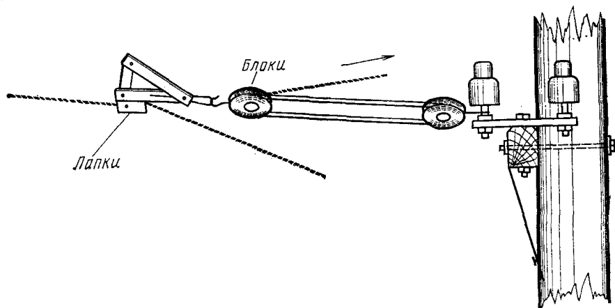
6.67. Натяжение проводов на конечных и контрольных опорах
