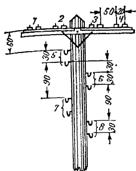
Профиль № 2а
