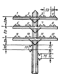
Профиль №4а
