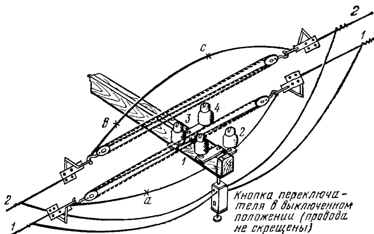
9.25. Устройство скрещивания на накладках (1-я операция)
