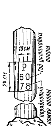
6.89. Нумерация фидерных и абонентских опор
