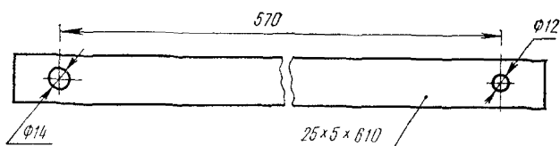
2.27. Подкос
