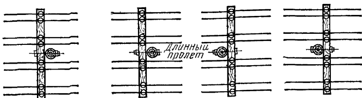
6.42. Расположение одинарных траверс при удлинненных пролетах
