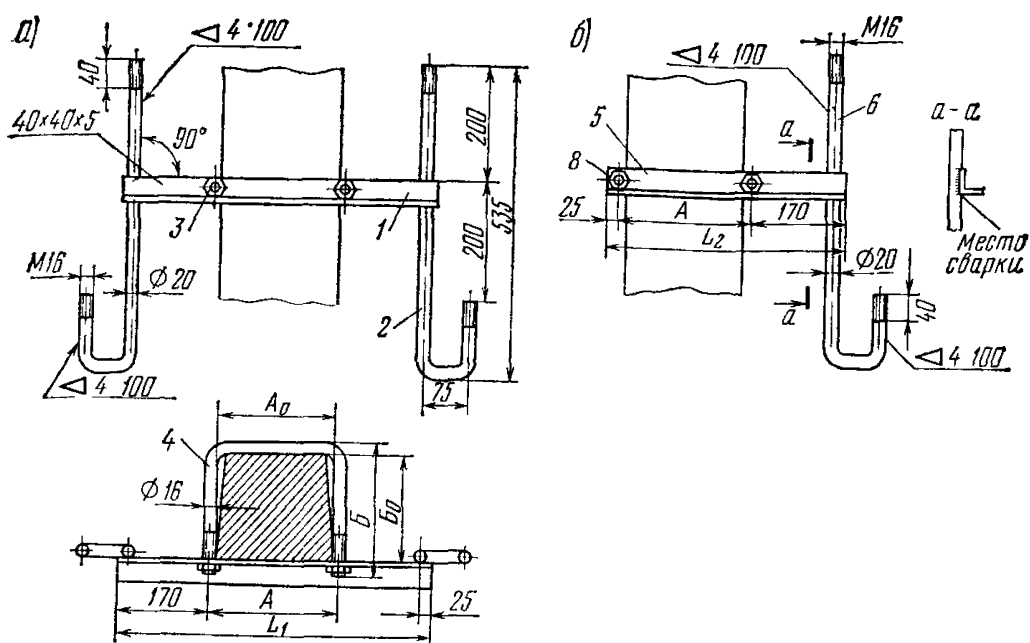
4.59. Арматура для подвески цепей РС на железобетонных опорах ВЛ прямоугольного сечения
