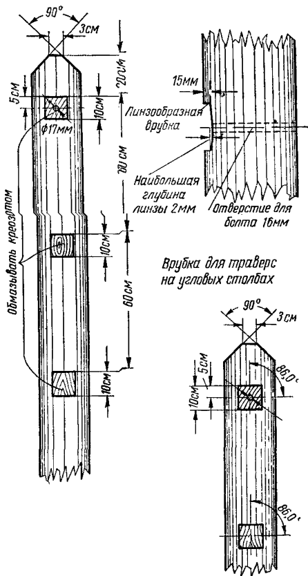
6.24. Затеска вершины опоры и врубки для траверс
