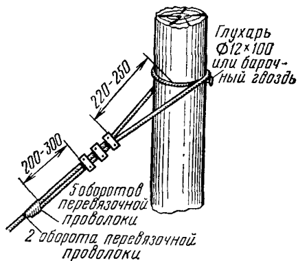
4.11. Крепление оттяжки из стального каната к опоре
