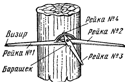
4.2. Общий вид измерителя вылета углов
