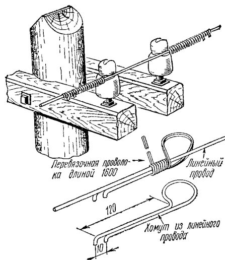
7.10. Двойное крепление проводов на траверсах
