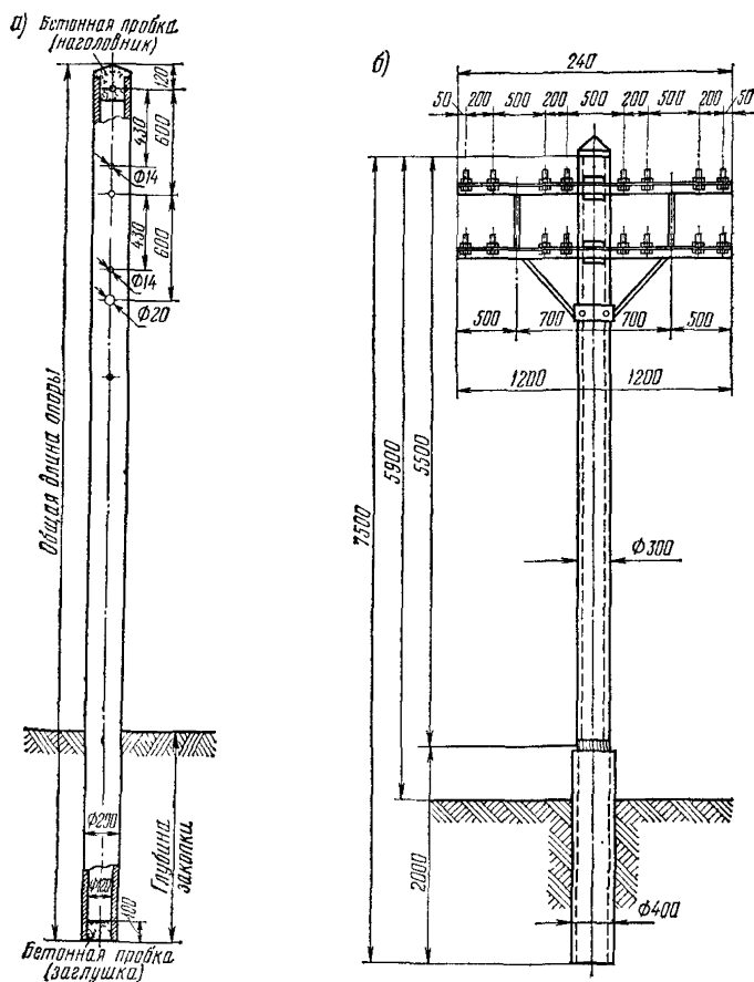
5.3. Круглые центрифугированные опоры: а) цилиндрические; б) конические
