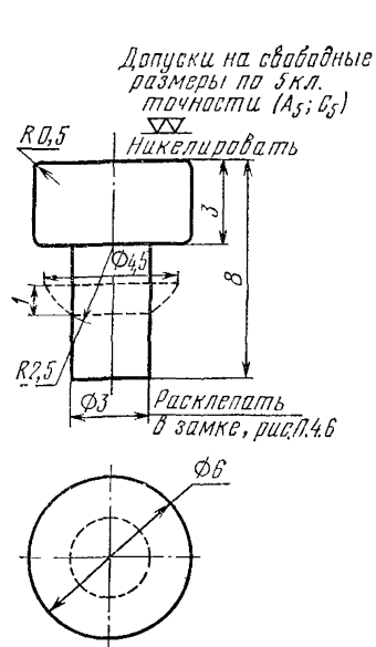
Рис. П.4.7 Специальная заклепка
