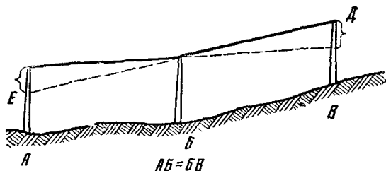
6.7. Определение величины уклона линии при тяжении проводов вверх
