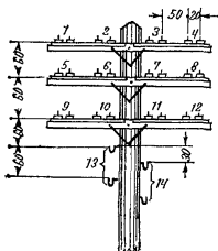
Профиль №4
