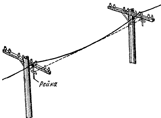
6.63. Регулирование проводов
