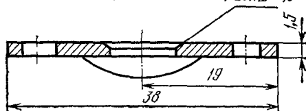
Рис. П.4.4. Замок
