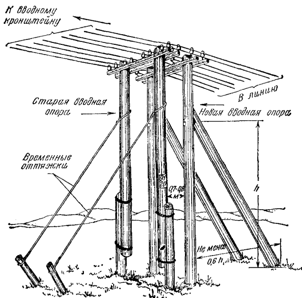
9.8. Замена оконечной полуанкерной опоры при установке новой опоры рядом со старой
