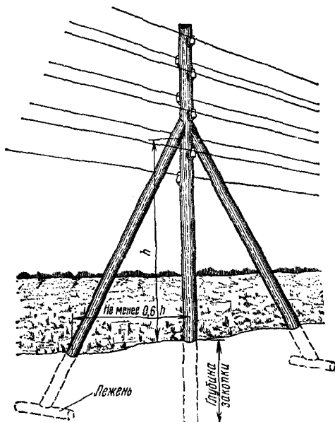
4.31. Усиленная опора
