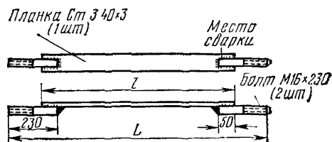
5.6. Хомут сварной
