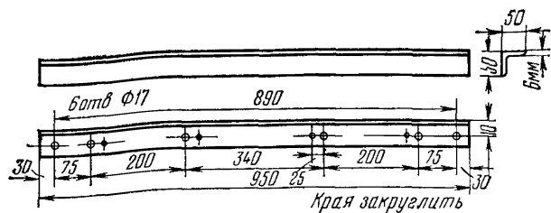
8 24. Траверса для кронштейна, применяемого на линиях РС или СТС
