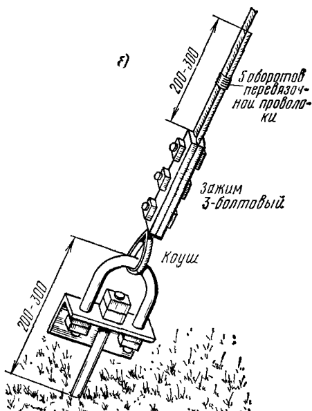
4.12. Способы крепления оттяжки из стального каната к якорному стержню
