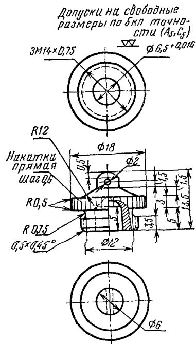
Рис. П.4.12. Головка зонда.
