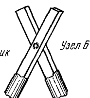
6.36. Способ установки опор при помощи «падающей стрелы»
