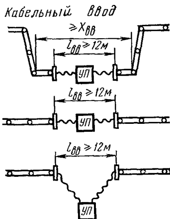
81. Схемы подходов линий к усилительным пунктам
