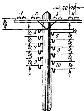
Профиль № 9
