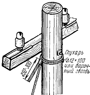
4.7. Начало заделки оттяжки на опоре
