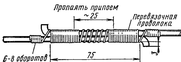
6.56. Спайка проводов
