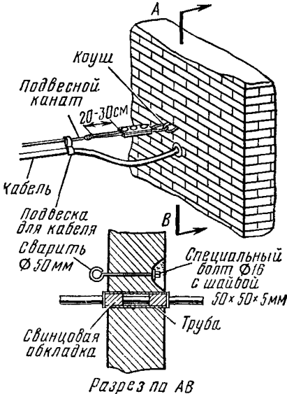
8.17. Ввод подвесного кабеля в здание
