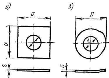
2.23. Шайбы:
