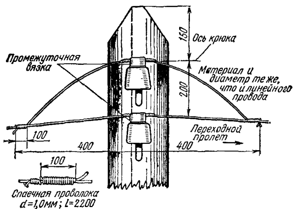
7.9. Двойное крепление проводов на крюках
