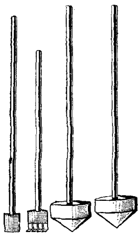
6.16. Бурофрез с ковшами двух диаметров
