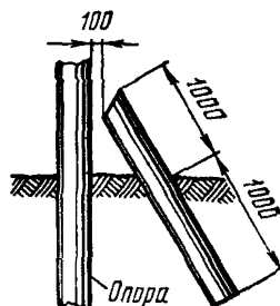
4.23. Отбойная тумба
