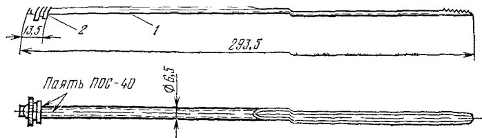
Рис. П.4.10. Зонд в сборе:
