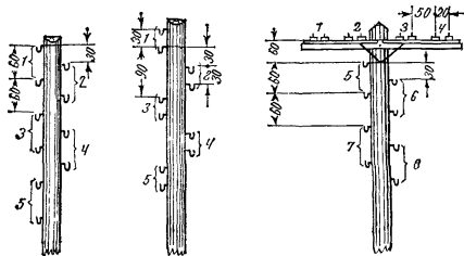
Профиль №1
