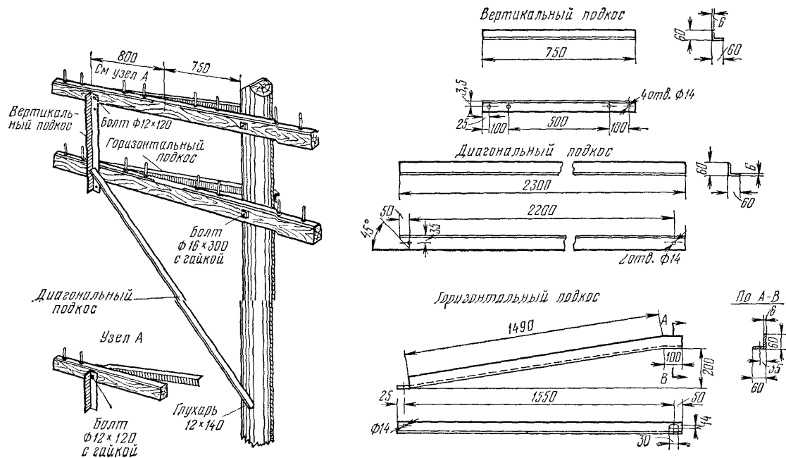
6.32. Неравноплечая траверса
