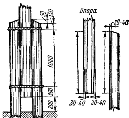
4.63. Укрепление опор двумя деревянными приставками
