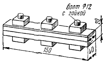
2.30. Трехболтовый зажим
