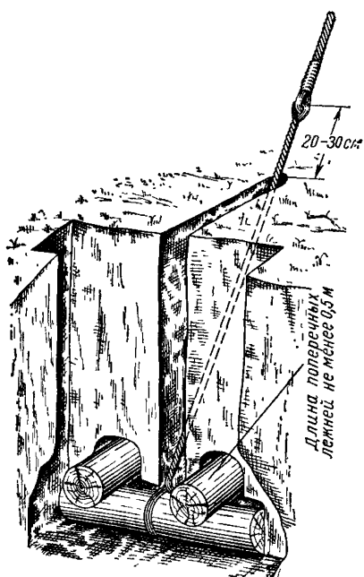
4.15. Заделка якорного лежня в слабых грунтах
