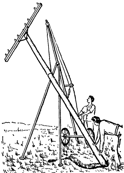
6.38. Подъем столба при помощи треноги
