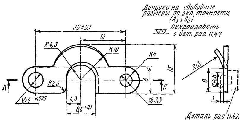
Разрез по А-В Фаска 0,5×45°
