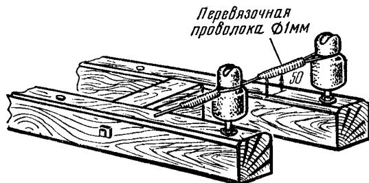
6.69. Оконечная заделка стальных проводов на двойных траверсах
