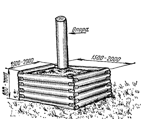
4.55. Устройство ряжа
