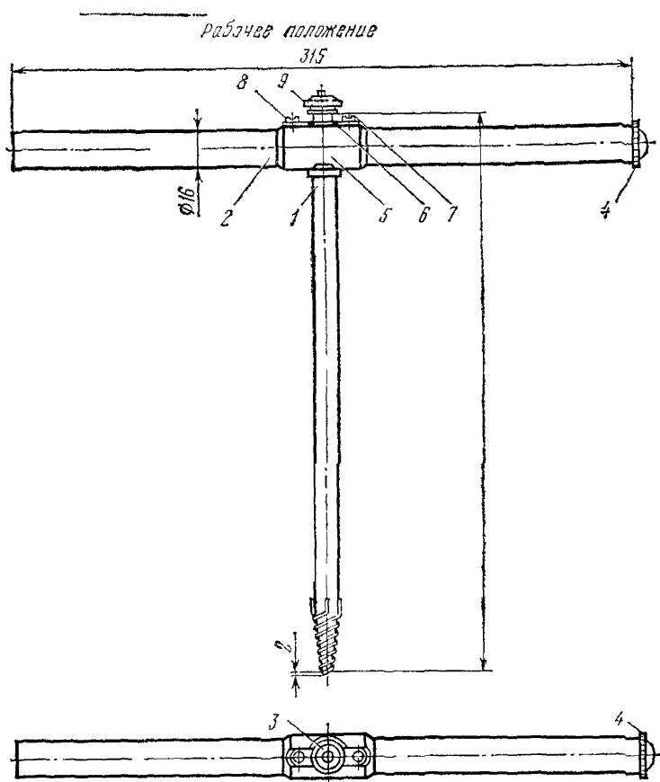
Рис. П.4.1. Пустотелый бурав в сборе:
