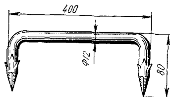
2.26. Скоба
