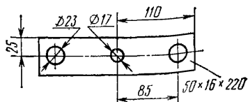
2.14. Накладка контрольная
