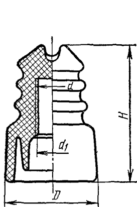
2.3. Изолятор трехшей- ковый типа РФО
