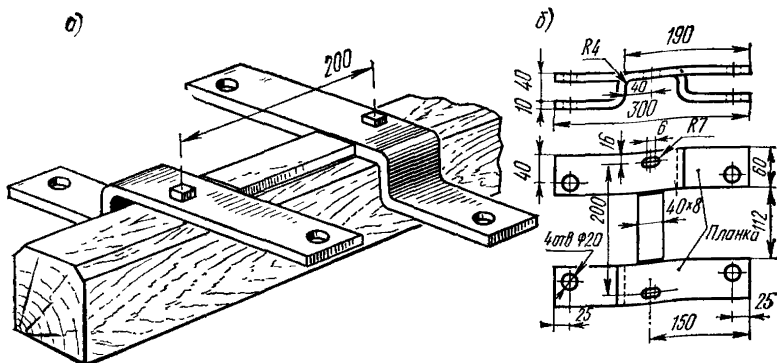
2.12. Накладка типа HD: а) общий вид; б) детали
