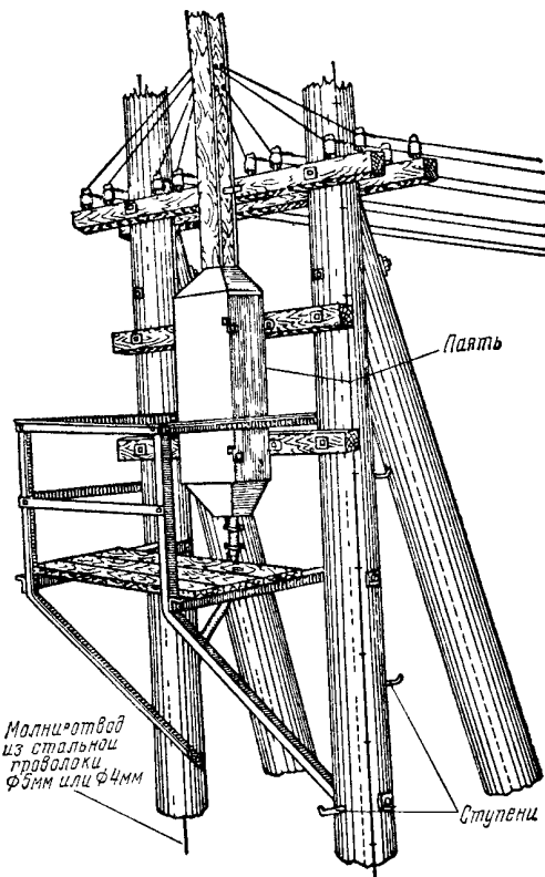
4.46. Кабельная опора полуанкерная
