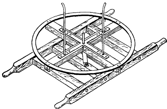
6.49. Тамбур ручной
