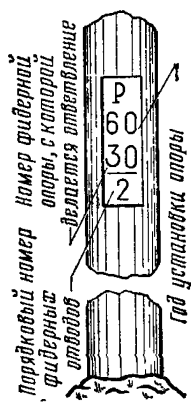
6.90. Нумерация опор фидерных отводов
