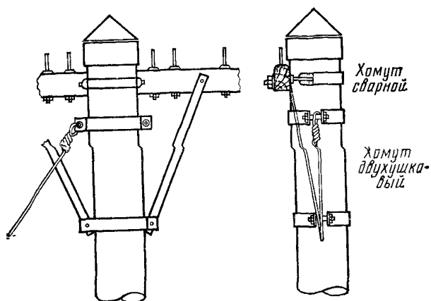
5.5. Крепление траверс и оттяжек к круглой опоре
