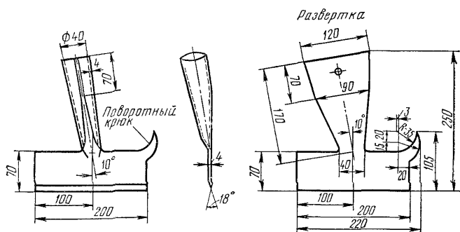
6.22. Окорочная лопасть
