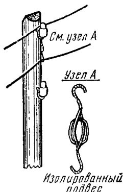
9.13. Замена крюка или изолятора на промежуточной опоре
