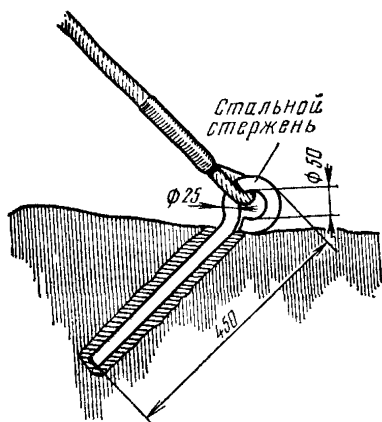
4.17. Крепление якоря в скалистых грунтах
