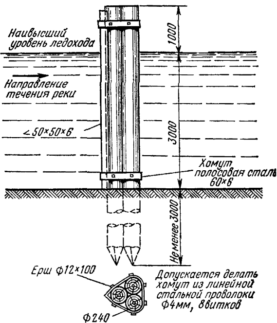
6.45. Кустовой ледорез
