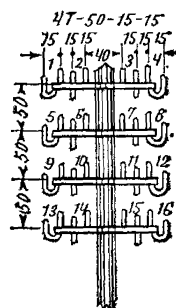
Профиль № 6а
