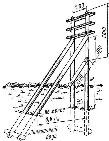
4.26. Полуанкерная опора, укрепленная подпорой
