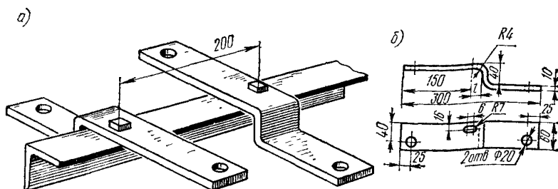
2.13. Накладки типов HC: а) общий вид; б) детали
