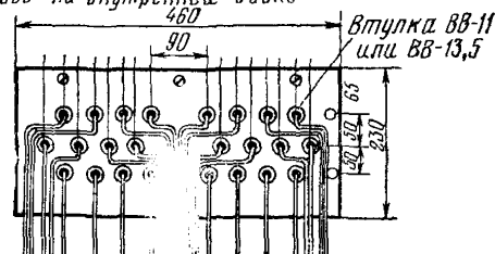
8.29. Расположение втулок и воронок на вводной коробке
