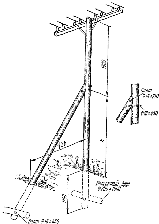
4.30. Противоветровая опора
