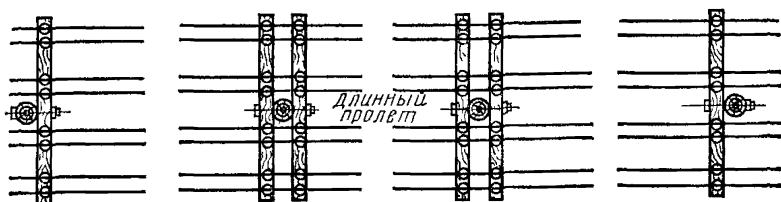
6.43. Расположение двойных траверс при удлинненных пролетах
