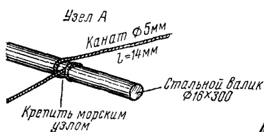
6.36. Способ установки опор при помощи «падающей стрелы»
