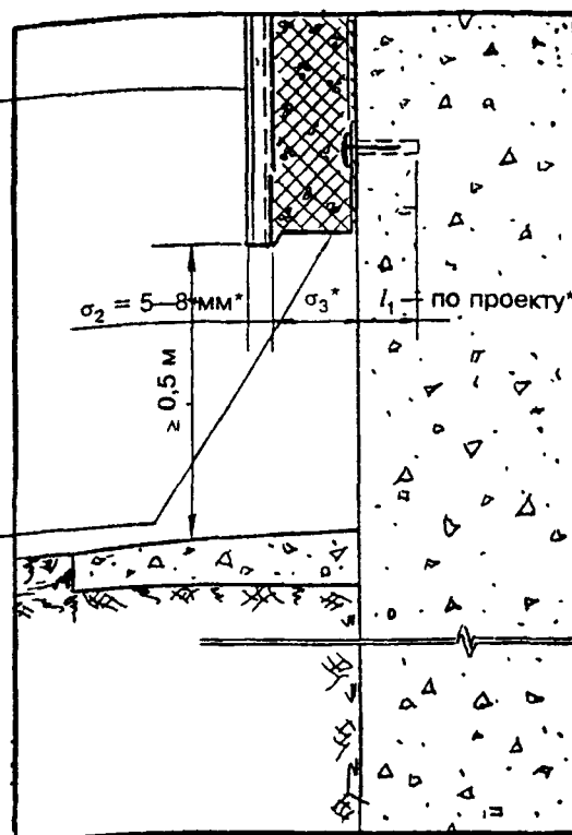
Рисунок А9 — Крепление теплоизоляционного слоя на нижней части стены
