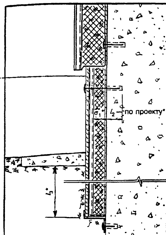
Рисунок А9 — Крепление теплоизоляционного слоя на нижней части стены
