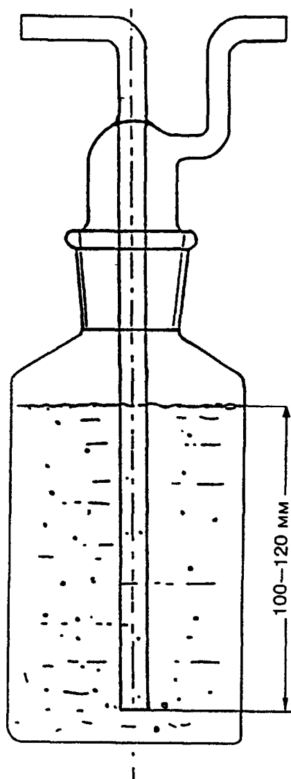
Рисунок 2 — Сосуд-смеситель
