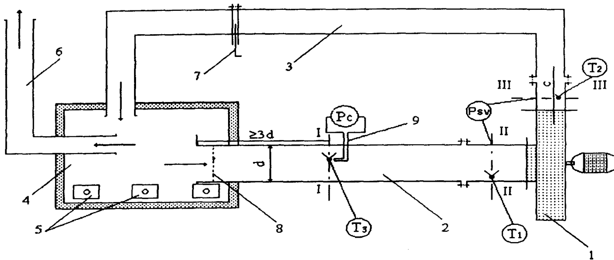
Рис. 1.1. Схема стенда для испытания вентиляторов:
