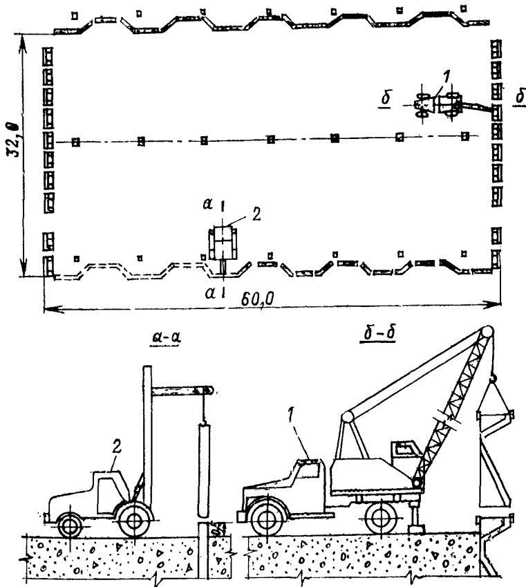
Схема раскладки опалубки межблочных швов
