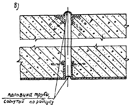
Рис. 18. Возможная конструкция деформационных швов.
