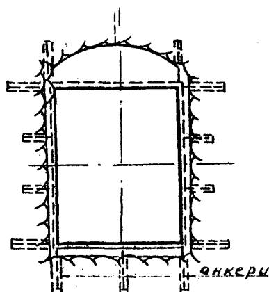
Рис. 5. Конструкция прианкеренной к породе стальной облицовки.
