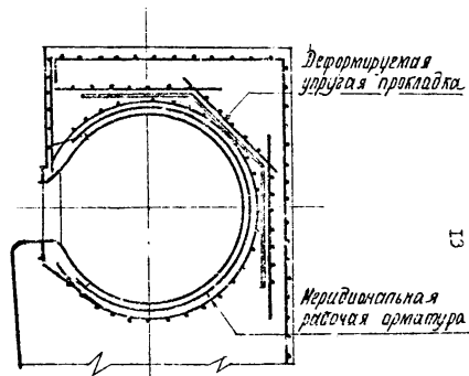
б. с деформируемой прокладкой
