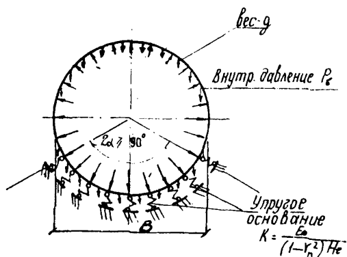
Рис.6 Расчетная схема открытого напорного трубопровода.
