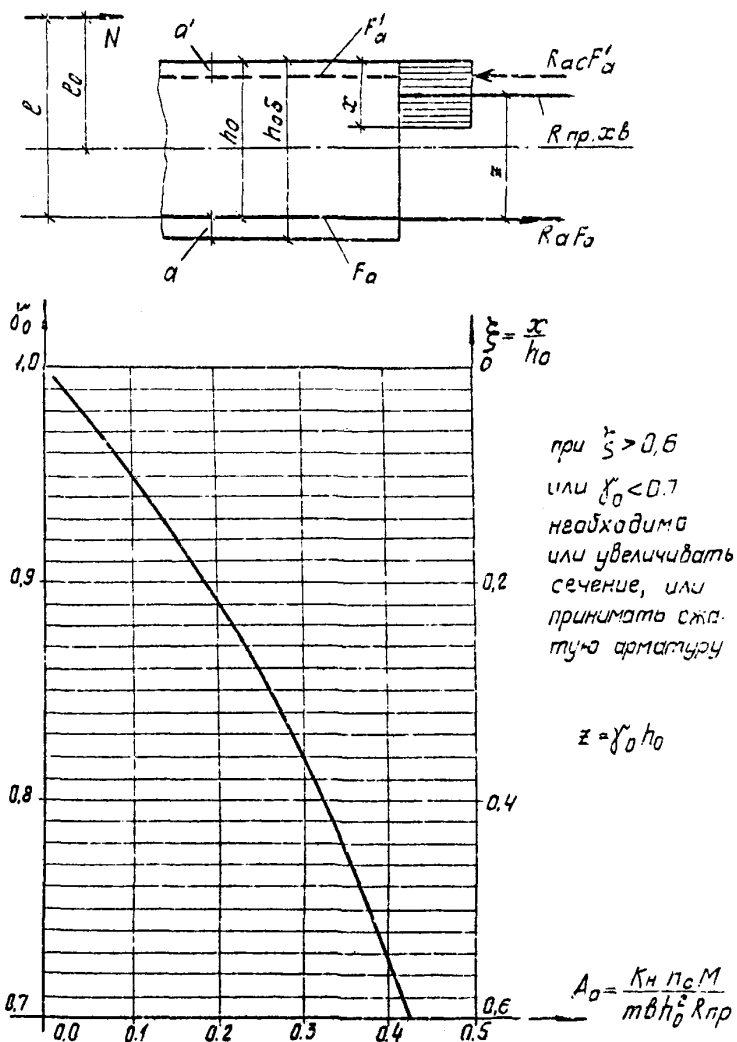
Рис. I. График для определения плеча внутренней пары сил железобетонного сечения.
