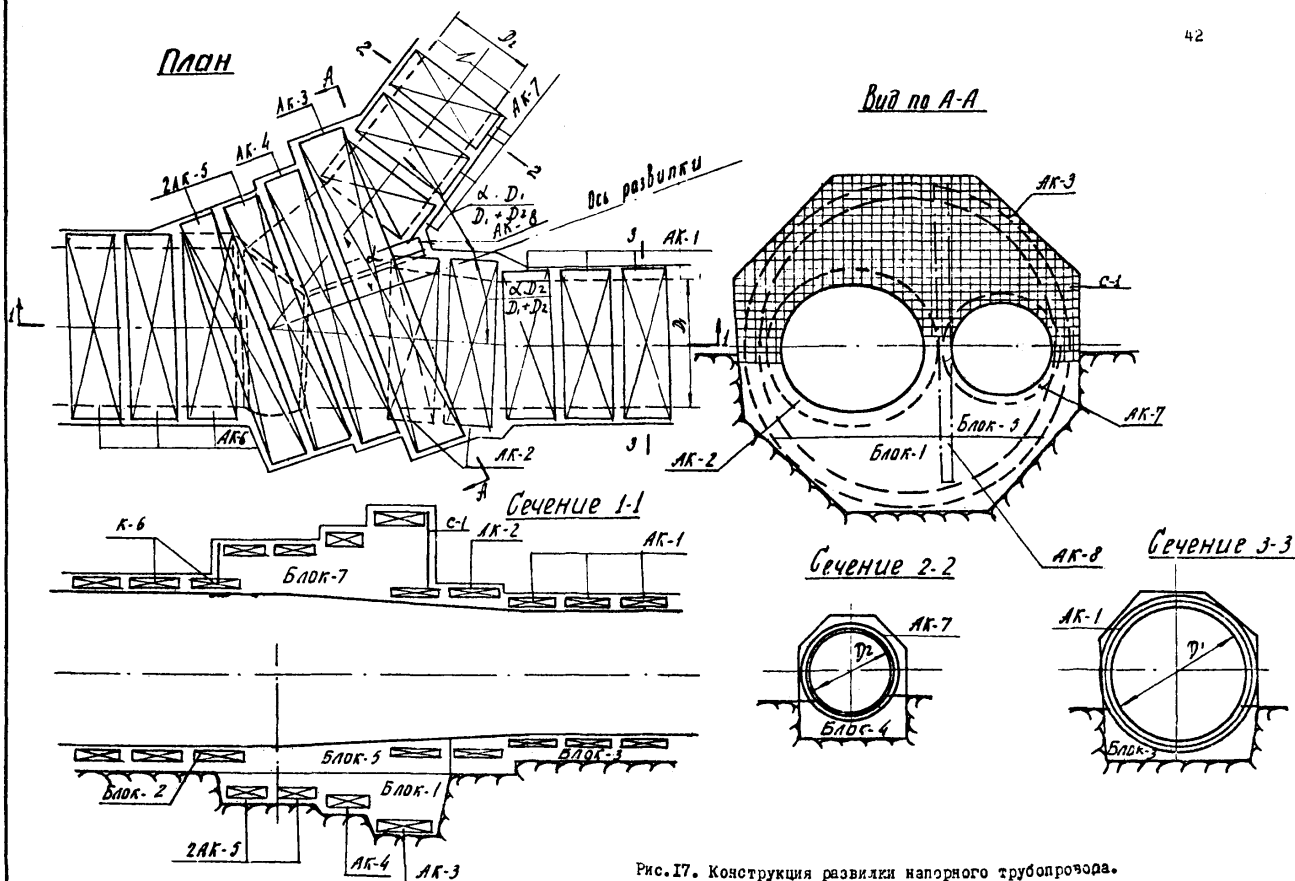
Рис.17. Конструкция развилки напорного трубопровода.
