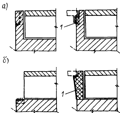
Рис. I4. I. Устройство прилива на опорной стенке для опирания переходных плит а - при наличии шкафной стенки; б - при отсутствии шкафной стенки I - приливка для опирания переходных плит
