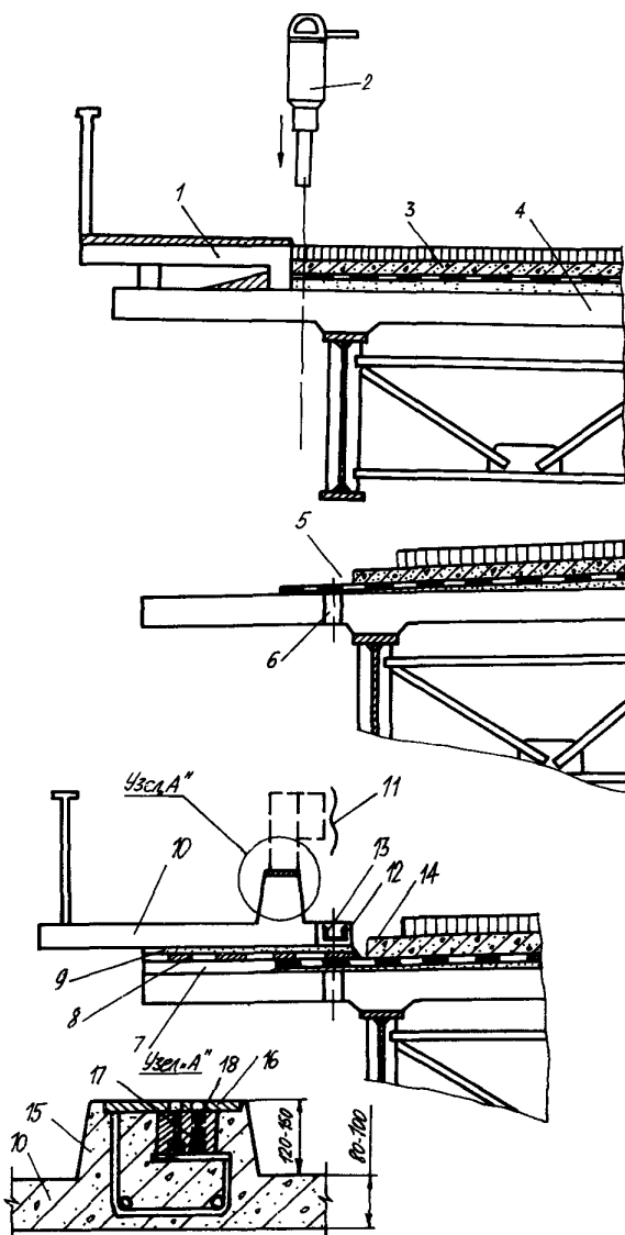
Рис.4.3. Замена тротуарного блока на новый с барьерным ограждением
