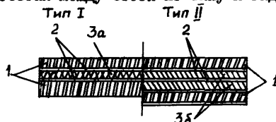
Рис.9.1. Конструкция гидроизоляции на основе битумно-латексной эмульсии
