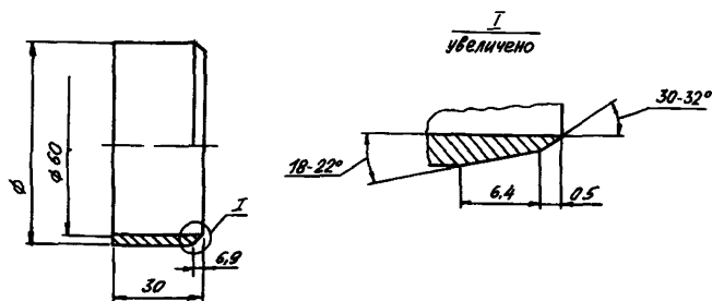
Рис.П.4.1.3. Шаблон для выручки образцов из мастики
