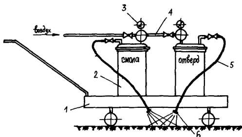
Рис.13.2.Схема распределителя материалов РД-601
