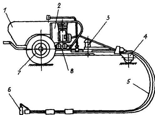
Рис.П.4.3.1.Схема установки для нанесения битумно-латексной мастики:
