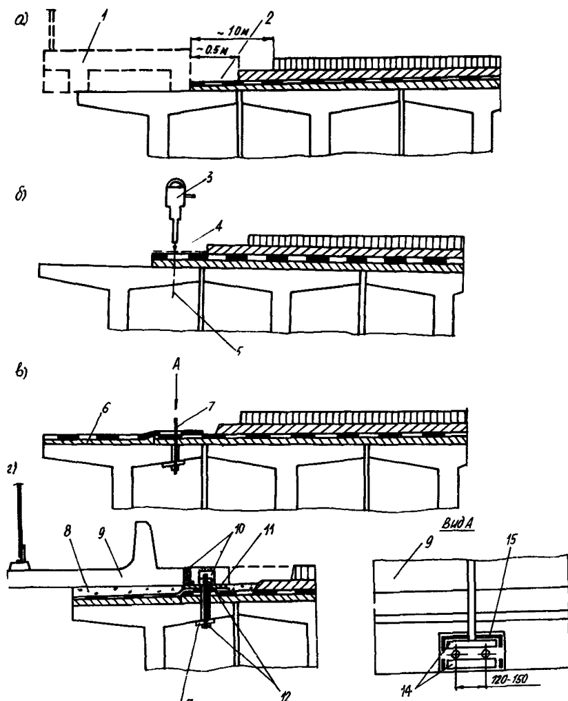
Рис.5.1. Замена тротуарного блока на новый с парапетным ограждением (а, б, в, г-этапы работы): 1-заменяемый тротуарный блок; 2-участок вырубki покрытия в защитного слоя; 3-сверлильная установка; 4-разметочный прямоугольник из рубероида; 5-ось отверстия под анкерный болт; 6-дополнительный выравнивающий слой и гидроизоляция под тротуар; 7-анкерный болт; 8-слой цементно-песчаного раствора под тротуар; 9-новый тротуарный блок; 10-закладные детали в нише тротуарного блока; 11-закладная анкерная пластинка; 12-гайка; 13-шайба; 14-отрезок стального профиля; 15-сварной шов
