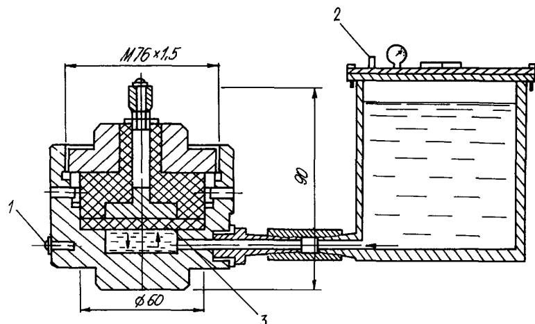
Рис.П.4.1.1. Прибор для определения водонепроницаемости
