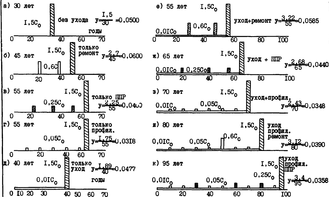
Рис. 1. Возможные схемы эксплуатации моста (учитывается лишь физический износ)
