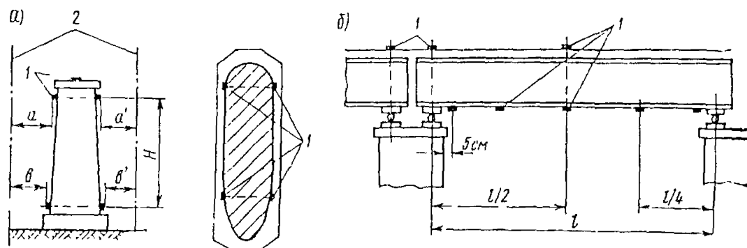
Рис. 12.1. Схема расположения закрепленных точек:
