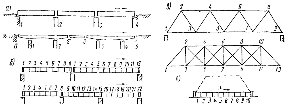
Рис 1.1 Схема обозначения элементов искусственного сооружения а — опор пролетных строений, б — диафрагмы и панелей, в — элементов сквозных ферм г — звеньев труб. Стрелкой показано направление хода километража для мостов.
