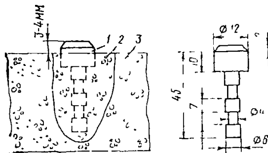
Рис. 122 Марка и ее закрепление в бетоне конструкции
