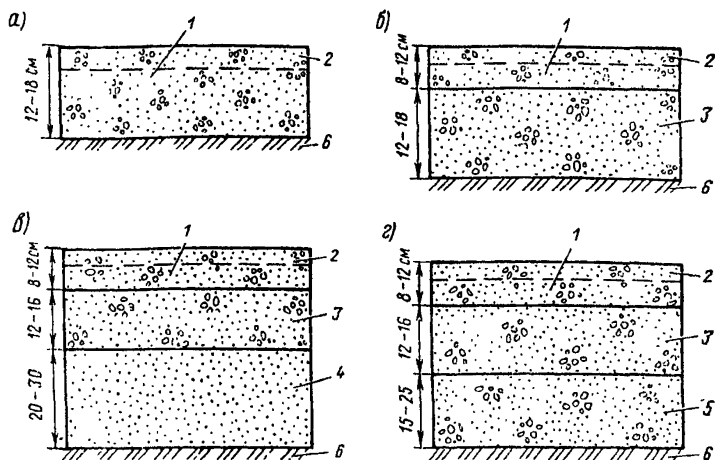
Рис. 1.2. Примеры конструкций дорожных одежд с гравийными покрытиями
