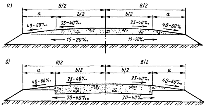
Рис. 1.1 Поперечные профили
