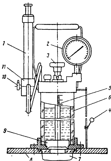
Рис. 1. Общий вид прибора КП-120
