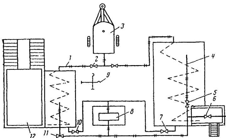
Рис. 1. Схема установки для приготовления обеспыливающих растворов
