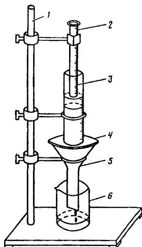
Рис. 1. Прибор для определения водостойкости лигносульфонатов технических
