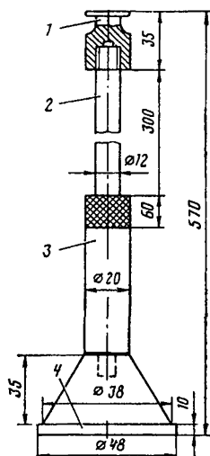
Рис. 2. Уплотнитель:
