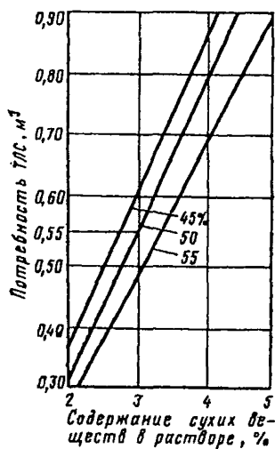
Рис. 2. Номограмма для определения количества ЛСТ при приготовлении 1 м³ раствора (цифры на прямых обозначают содержание сухих веществ в ЛСТ)
