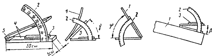
Рис. 3.1. Угломер и его установка при замеры углов захвата \varphi , резанья \gamma и наклона \beta : 1 — отвал автогрейдера; 2 — сектор; 3 — уровень; 4 — рейка; 5 — шарнир
