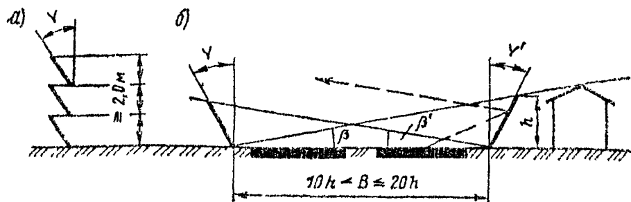
Рис 16.6 Схема ступенчатого шумоотражающего барьера с основными геометрическими размерами:
