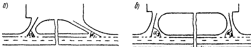
Рис 14.3 Схемы подъездов к сооружениям обслуживания, располагаемым в придорожной полосе
