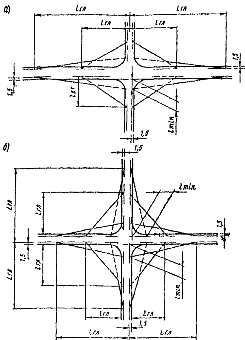
Рис 6.1 Схемы определения видимости на пересечениях в одном уровне а — при пересечении дорог разных категорий, б — при пересечении равнозначных дорог
