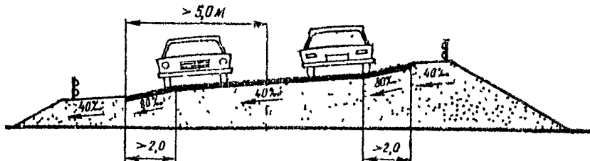
Рис. 4.1. Схема устройства ступенчатого виража на кривых малого радиуса
