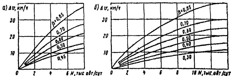
Рис. 1.10. Влияние интенсивности и состава движения на снижение средней скорости:
