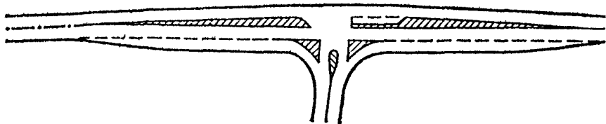
Рис 6.10 Направляющие островки на примыкании в одном уровне
