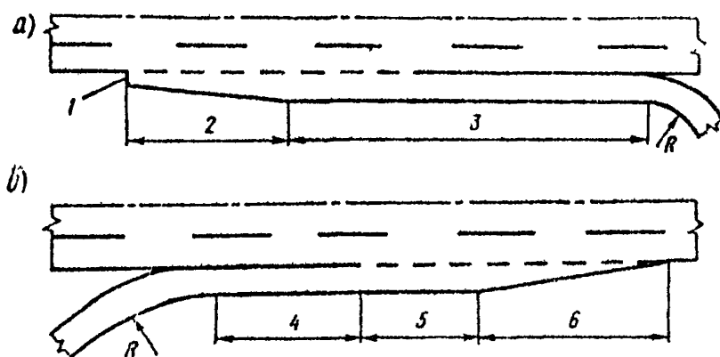
Рис 77 Элементы полос торможения (а) и разгона (б).
