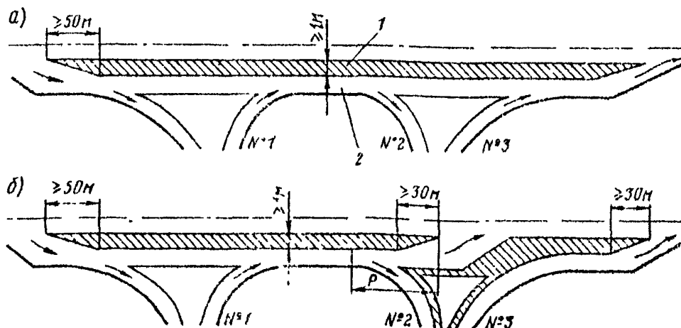
Рис 7.3 Конструкция боковой разделительной полосы на развязке «клеверный лист»
