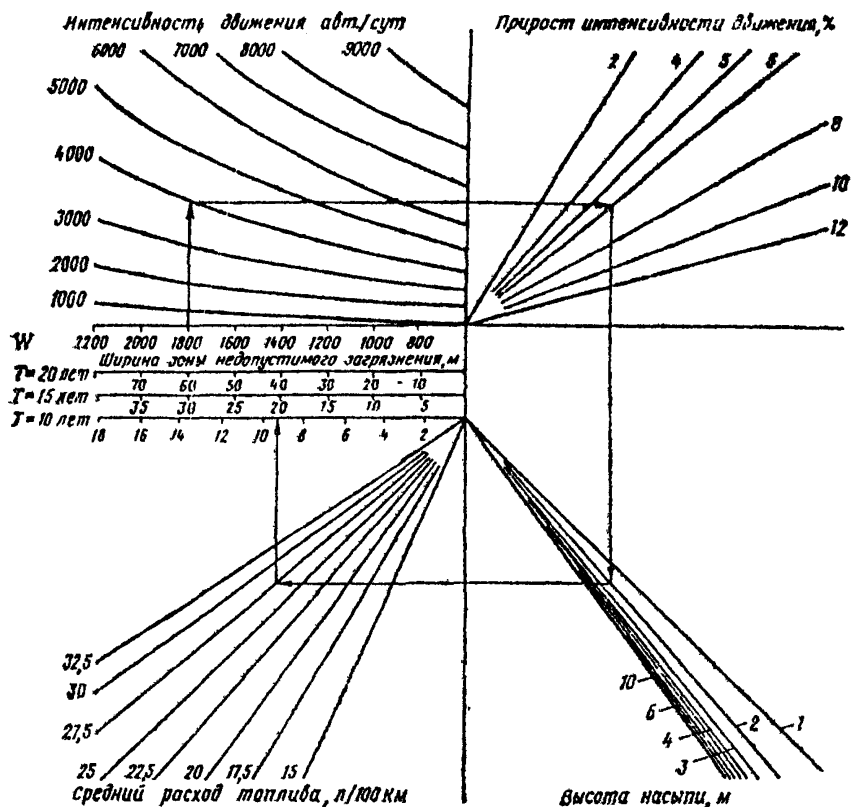
Рис. 16.10. Номограмма для расчета ширины зоны, в пределах которой содержание свинца в почве превышает его предельно допустимую концентрацию
