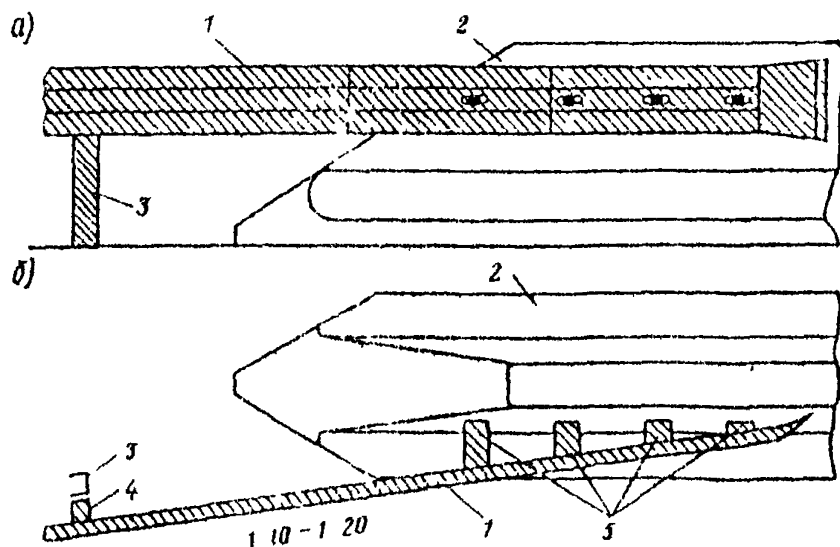
Рис 11.2 Сопряжение барьерного ограждения с парапетным а — профиль, б — план, 1 — планка, 2 — парапет, 3 — стойка, 4 — амортизатор, 5 — стойки упоры
