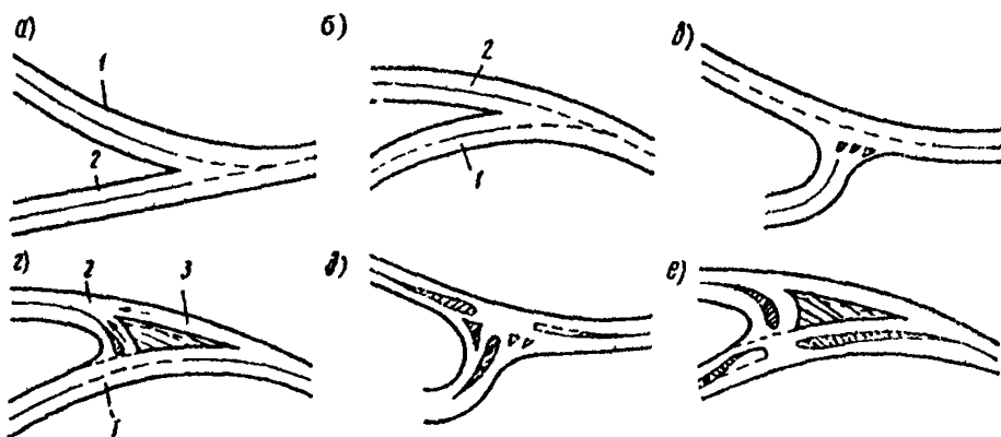
Рис 6.6 Рекомендуемые схемы планировки пересечений в одном уровне на обходе городов
