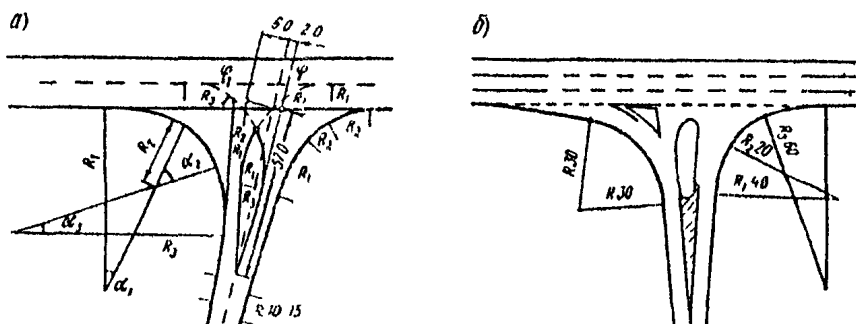
Рис 612 Расположение островков на второстепенной дороге а — схема размещения островка б — выделение островка разметкой
