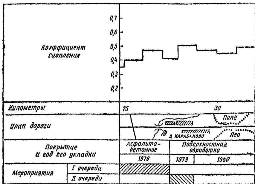
Рис. 2.7. Линейный график коэффициентов сцепления
