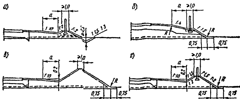
Рис. 16.8. Рекомендуемые поперечные профили земляного полотна для размещения шумозащитных сооружений:
