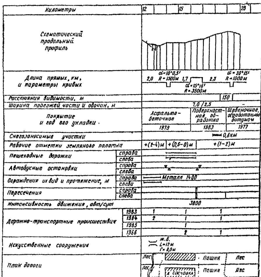
Рис 21. Линейный график дороги
