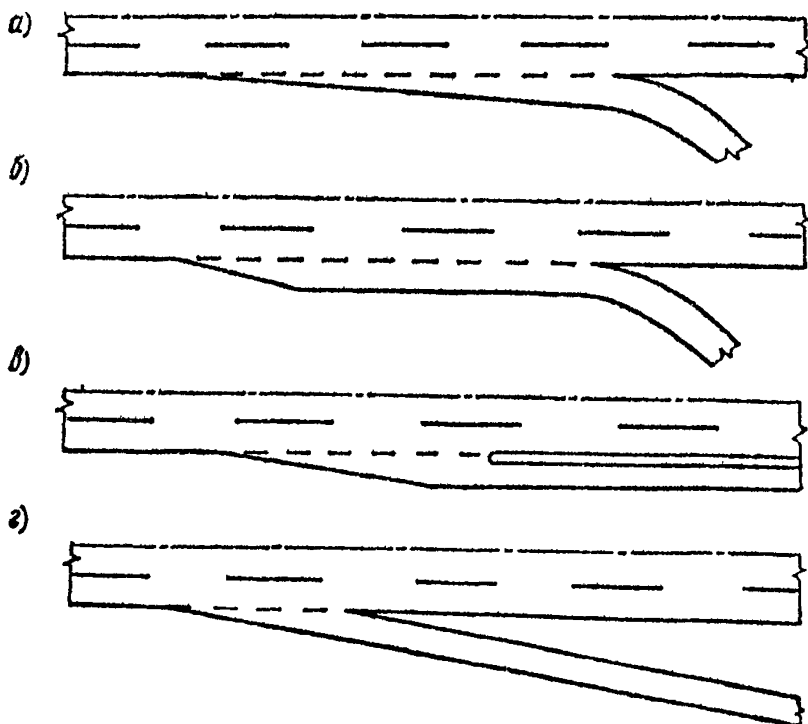
Рис 78 Типы переходно скоростных полос
