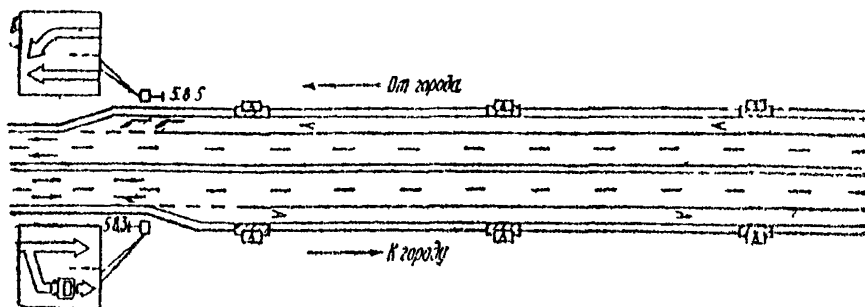
Рис. 133 Схема движения при устройстве дополнительной полосы только для автобусов
