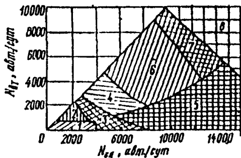
Рис 6 2. Номограмма для выбора типа планировочных решений пересечений.
