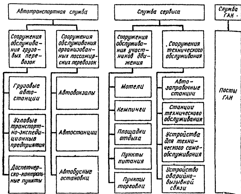
Рис 14.1 Схема сооружений для обслуживания транспортных средств и участников движения на автомобильных дорогах
