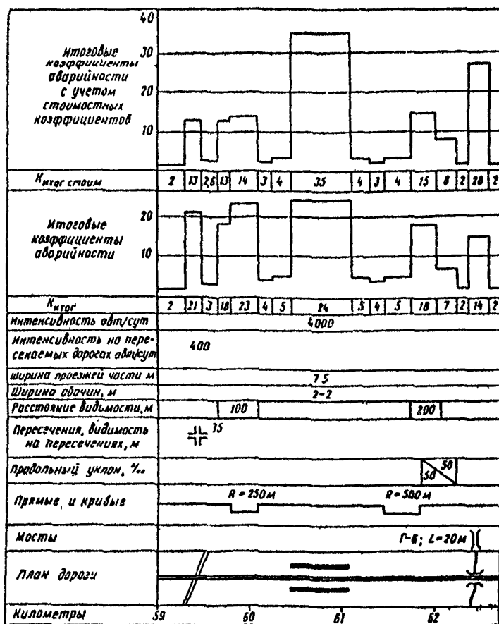
Рис. 13. Уточнение графика итоговых коэффициентов аварийности введенным поправочных коэффициентов тяжести ДТП
