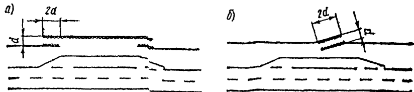
Рис. 16.9. Схемы расположения контрбарьера (а) и дубль-барьера (б) у остановки общественного транспорта в населенном пункте
