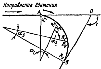
Рис. 6 4 Схема для расчета коробовой кривой
