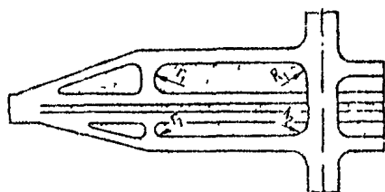
Рис 76 Схема планировки развязки обжатый «клеверный лист»
