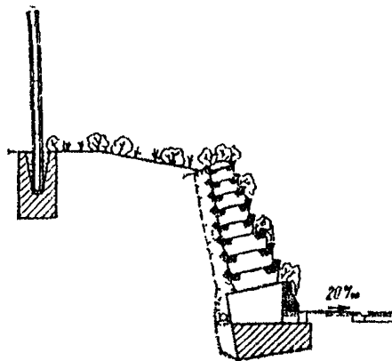
Рис. 16.1 Пример образования сложной для службы эксплуатации зоны между двумя шумозащитными сооружениями
