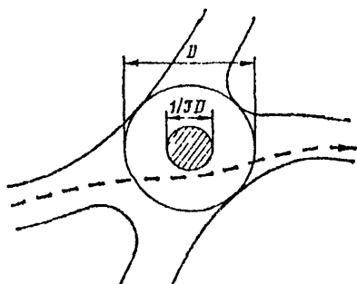
Рис 6 17. Улучшение условий движения на пересечении путем устройства островков небольшого диаметра
