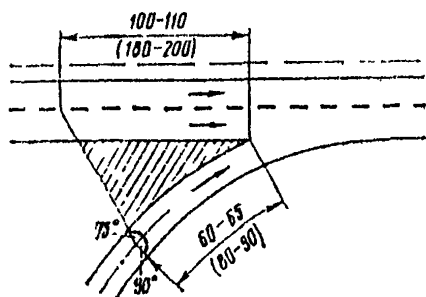
Рис 75 Параметры треугольника видимости на выходных участках съездов транспортных развязок
