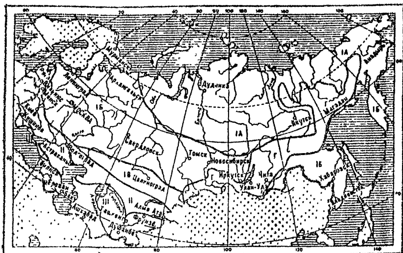
Рис. 1.7. Районирование территории СССР по условиям движения автомобилей.
