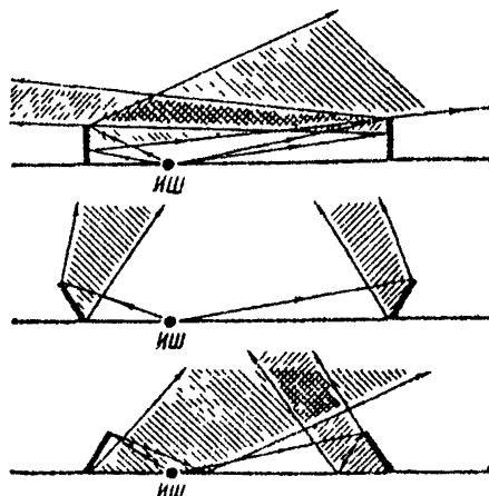
Рис 165 Ограждение звука от барьеров при различном их наклоне ИШ — источник шума
