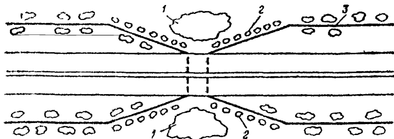
Рис. 16.11 Схема устройства перехода для диких животных. 1 — растения привлекающие животных, 2 — декоративный кустарник, скрывающий ограждение, 3 — ограждение
