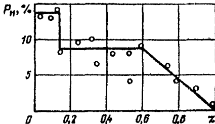
Рис 2.4 Зависимость темпов прироста интенсивности движения P_n от коэффициента загрузки z
