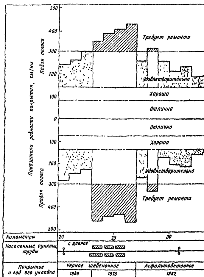
Рис 2.6 Линейный график ровности
