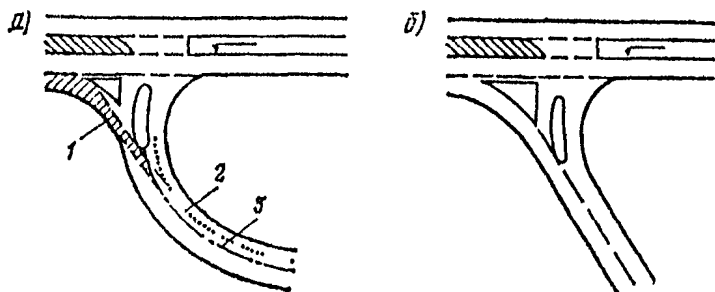
Рис 69 Зрительное перекрытие островками неправильного направления движения:
