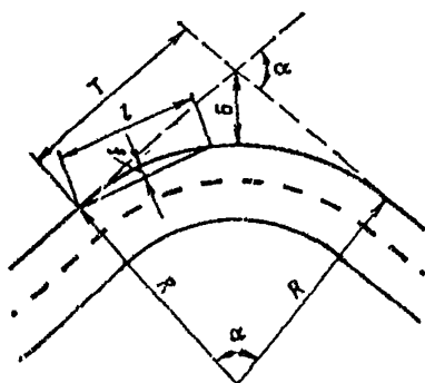
Рис 25 Схема закругления в плане и, элементы для определения радиуса
