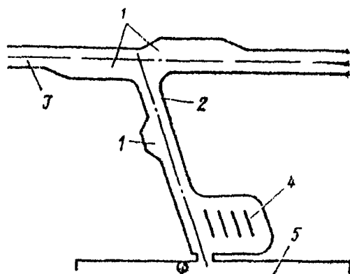
Рис 138. Схема подъезда к тупиковому заготовительному пункту:
