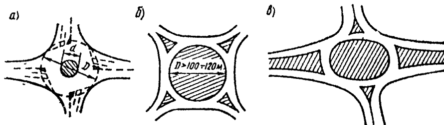
Рис 6 16 Планировочные схемы кольцевых пересечений
