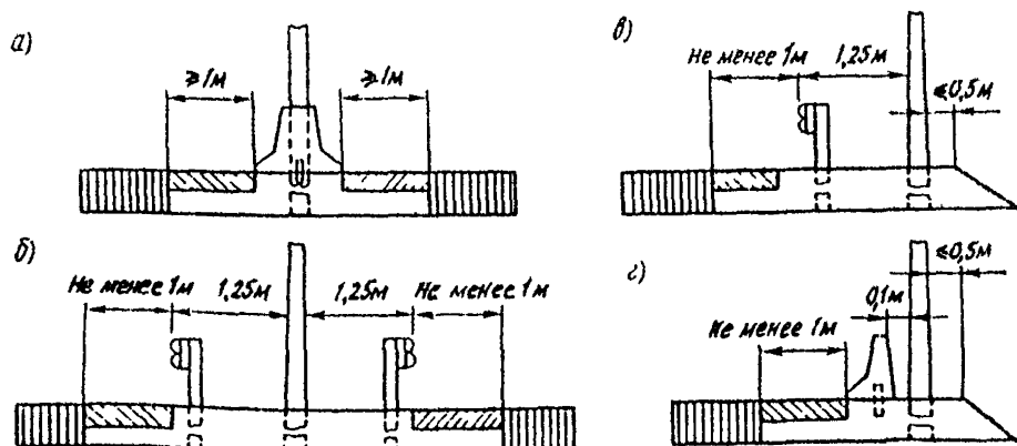
Рис 15.2. Схема установки опор освещения и ограждения на разделительной полосе (а, б) и обочине (в, г)
