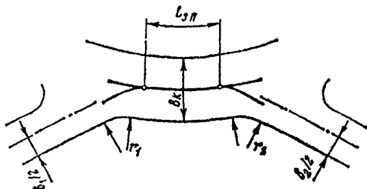
Рис. 618 Схема к расчету диаметра центрального островка на кольцевом пересечении.
