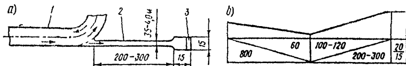
Рис 51 Схема аварийного съезда:
