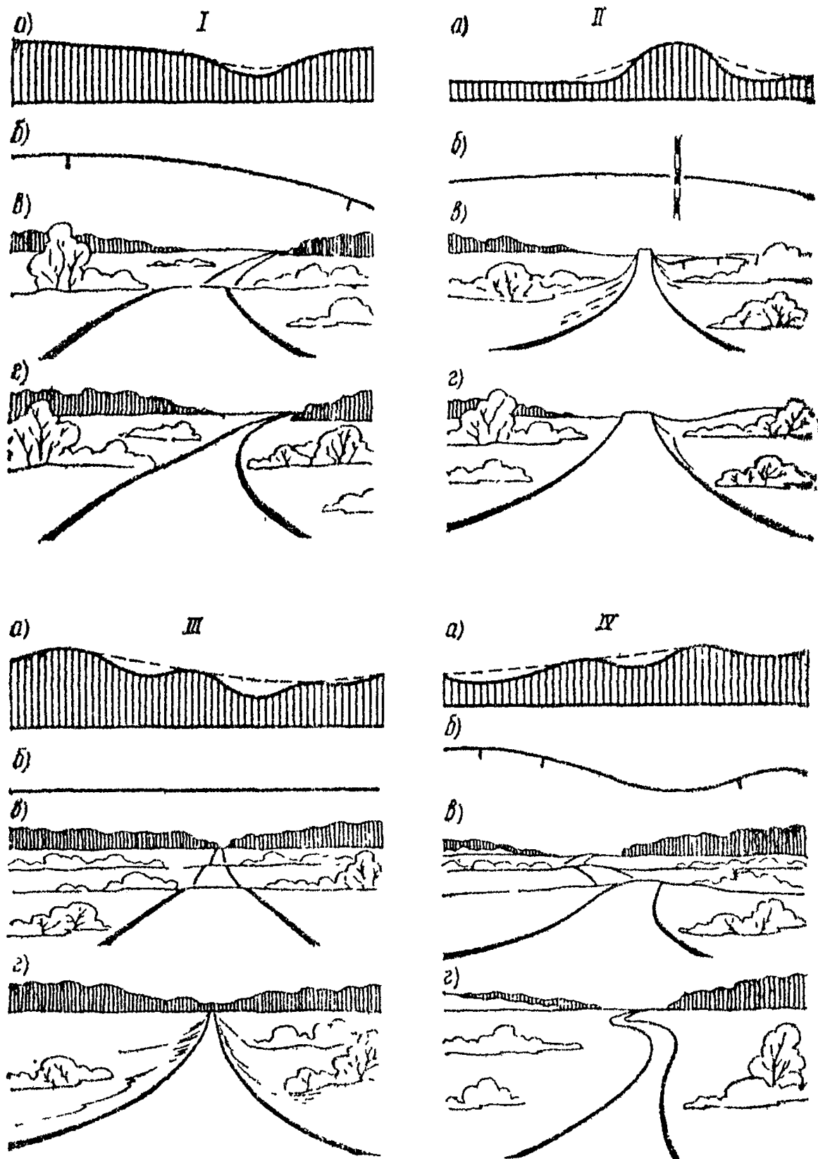
Рис 34 Типичные примеры нарушения план I — короткие вогнутые участки, II — крутые выпуклости продольного профиля, III — короткие горизонтальные кривые, IV — короткие прямые а — продольный профиль, б — план трассы, в — перспективный вид до улучшения пла н-профиля
