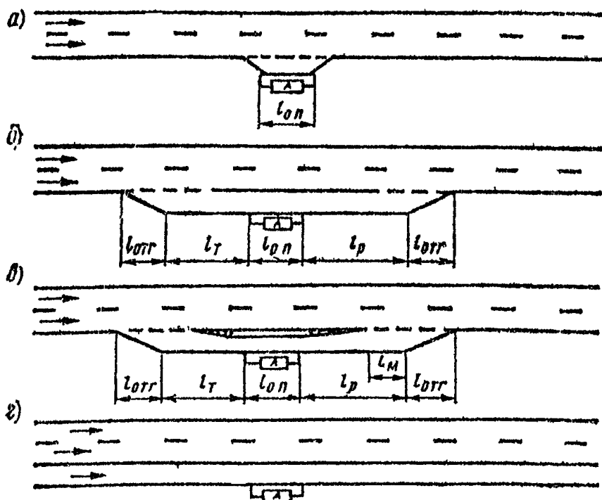
Рис. 131 Варианты планировочных решений в зоне автобусных остановок для отделения маршрутных автобусов от потоков автомобилей: а — простой «карман», б — переходно-скоростные полосы, в — переходно-скоростные полосы с разделительным островком; г — дополнительная полоса для автобусов
