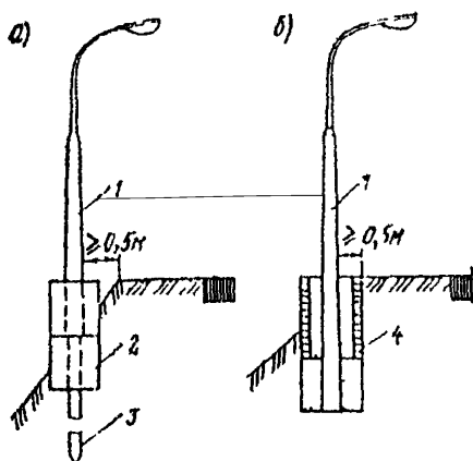
Рис 15.1. Схемы заделки в грунт опор освещения:
