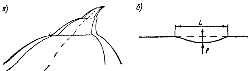
Рис. 3.2. Образование зрительных провалов на участках прямых с вертикальными кривыми
