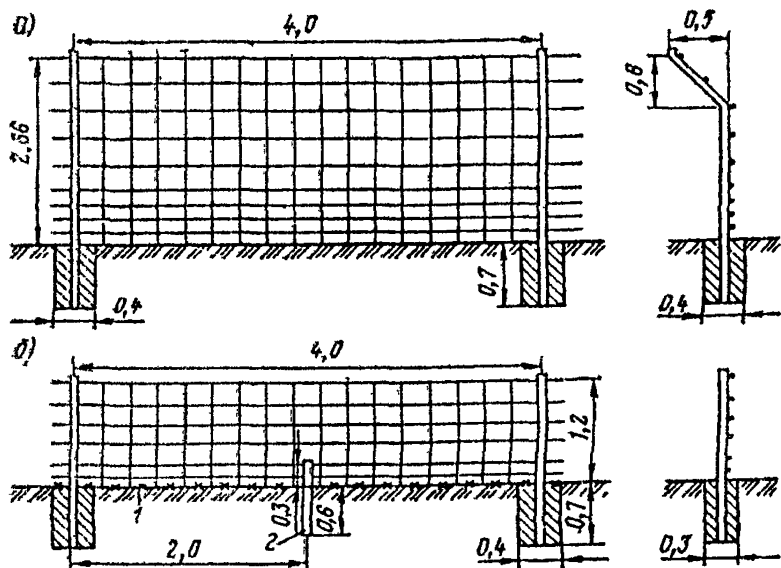
Рис. 16.12 Ограждения, предотвращающие выход на дорогу крупных копытных животных (а), кабанов (б).
