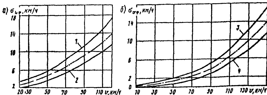
Рис. 1.9 Зависимость среднего квадратического отклонения \sigma_{vf} от максимальной скорости
