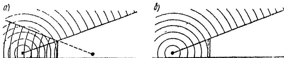
Рис. 164. Схема распространения шума при устройстве барьера а — шумоотражающего, б — шумопоглощающего
