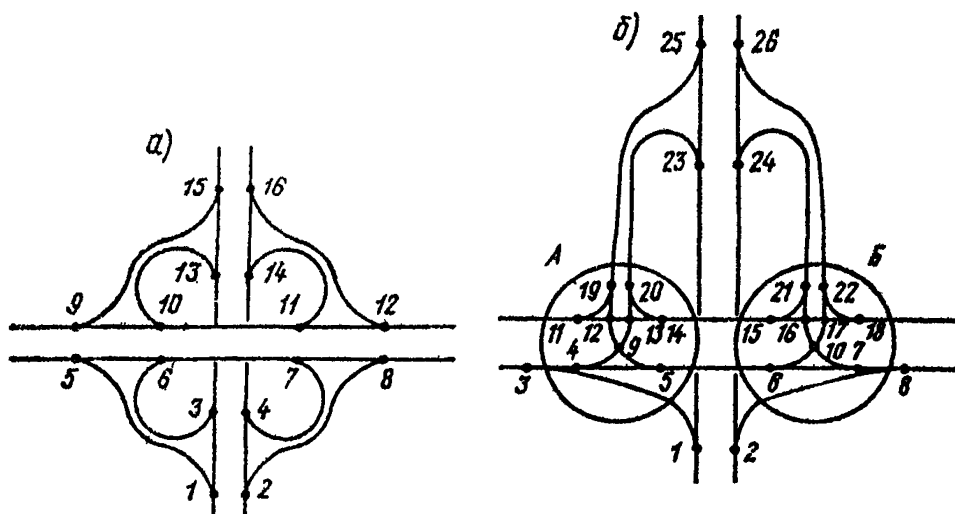
Рис. 1.5. Схема конфликтных точек на транспортных развязках: а — полная транспортная развязка (2, 3, 5, 7, 10, 14, 12, 15 — точки разделения потоков; 1, 8, 9, 16, 4, 6, 11, 13 — точки слияния потоков); б — неполная транспортная развязка (А и Б — узлы, оцениваемые как пересечения в одном уровне по табл. 1.13, 1, 2, 3, 8, 23, 24, 25, 26 — точки, оцениваемые по табл. 1.18)
