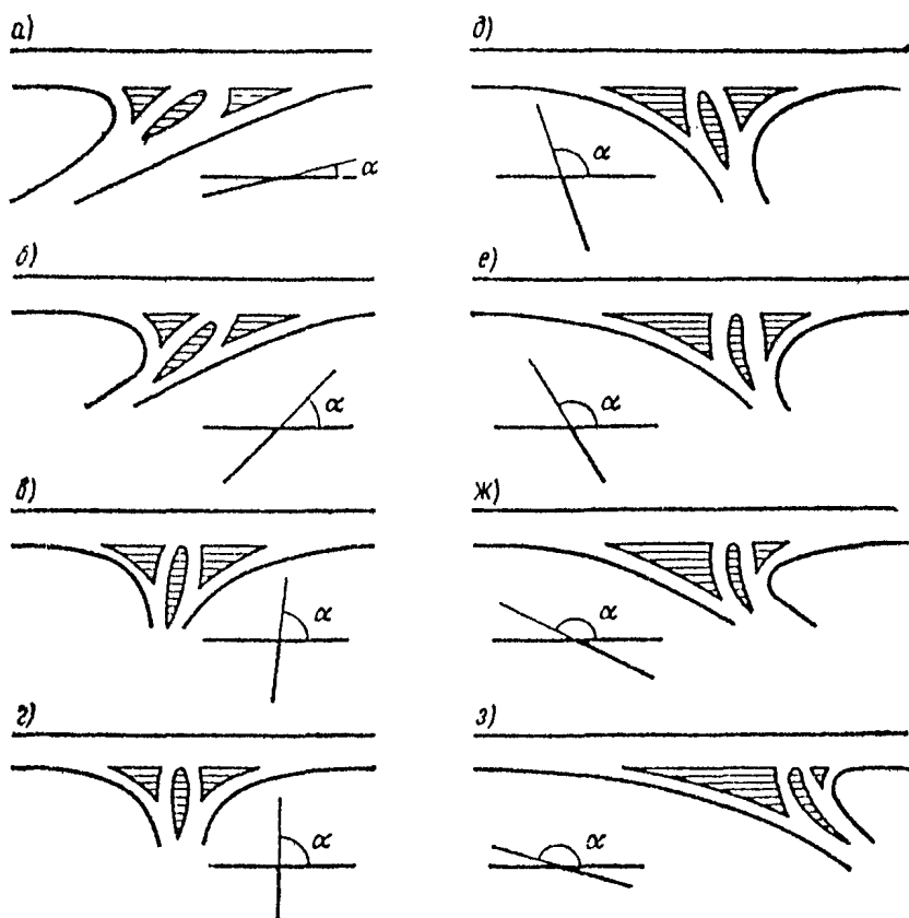
Рис 6.14 Изменение планировки в зависимости от угла пересечения дорог: а — \alpha < 30^\circ , б — \alpha = 30-45^\circ , в — \alpha = 50-75^\circ , г — \alpha = 90^\circ , д — \alpha = 115^\circ , е — \alpha = 135^\circ , ж — \alpha = 160^\circ , з — \alpha > 150^\circ
