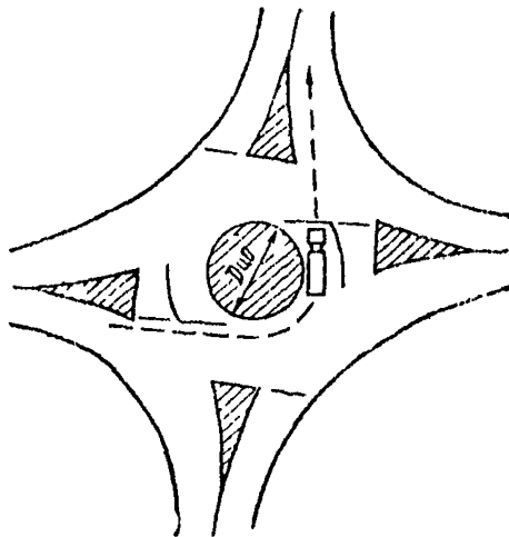
Рис. 619 Схема расположения автопоезда в зоне ожидания на кольцевой проезжей части
