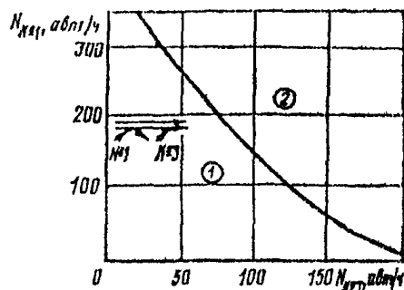
Рис 74 Области применимости различных видов планировки боковой разделительной полосы
