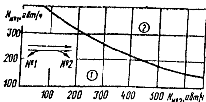
Рис 7.1. Диаграмма применимости различных типов левоповоротных съездов
