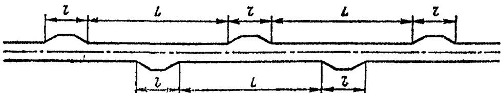
Рис. 13.6 Расположение дополнительных обгонных полос / в плане на участке дороги с интенсивным движением тракторов
