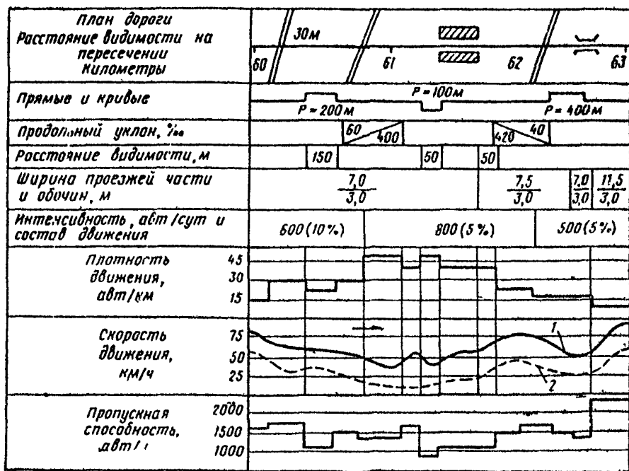
Рис 2.2. График изменения режима движения по длине дороги: 1 — легковые автомобили, 2 — грузовые автомобили, в скобках указана доля тяжелых грузовых автомобилей в потоке
