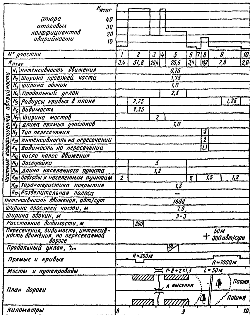
Рис. 1.2. Пример графика итоговых коэффициентов аварийности
