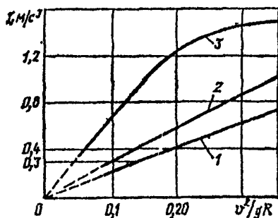
Рис. 4.2 График для определения расчетного нарастания центростремительного ускорения
