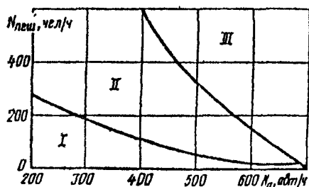
Рис 10.1 Области применения пешеходных переходов различных типов. I — нерегулируемые переходы, II — светофорное регулирование, III — подземные переходы
