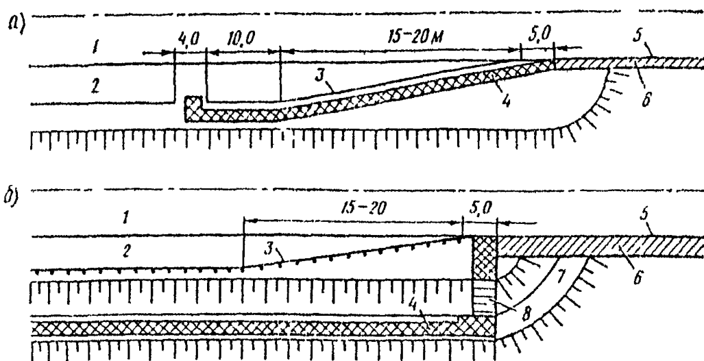
Рис 11.1 Схема расположения ограждений и пешеходных дорожек на подходах к мостам
