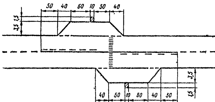
Рис. 10.2 Оборудование автобусных остановок в населенных пунктах
