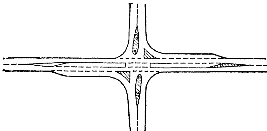
Рис 6.15 Выделение островков на проезжей части разметкой
