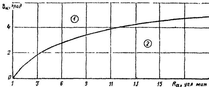
Рис 3.3 График для определения зрительной плавности дороги 1 — зрительная плавность не обеспечена, 2 — зрительная плавность обеспечена
