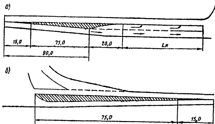
Рис 6.13 Расположение островков на главной дороге а — ченоповоротный островок, б — направляющий островок
