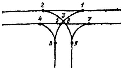
Рис. 14 Схема конфликтных точек на примыканиях автомобильных дорог в одном уровне
