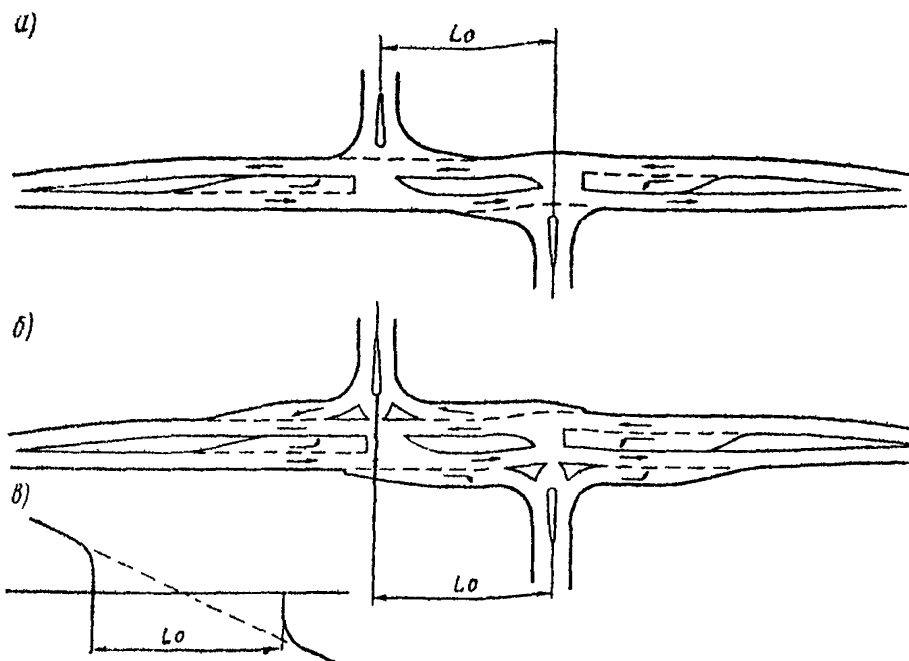
Рис. 6.7. Перестройка пересечения на два смещенных примыкания а — без переходно-скоростных полос, б — с переходно-скоростными полосами, в — схема изменения пересечения
