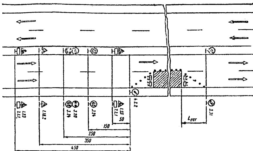
Рис. 3.10. Организация движения и ограждение места дорожных работ, выполняемых на дополнительной полосе на подъеме
