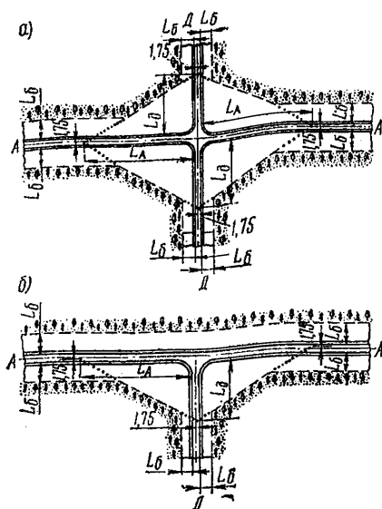
Рис. 6. Схемы обеспечения видимости:
