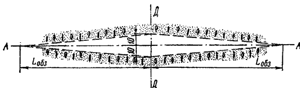
Рис. 7. Схема видимости по главной дороге и обзорности с второстепенной
