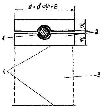
Рис 2 Шарнирное устройство:
