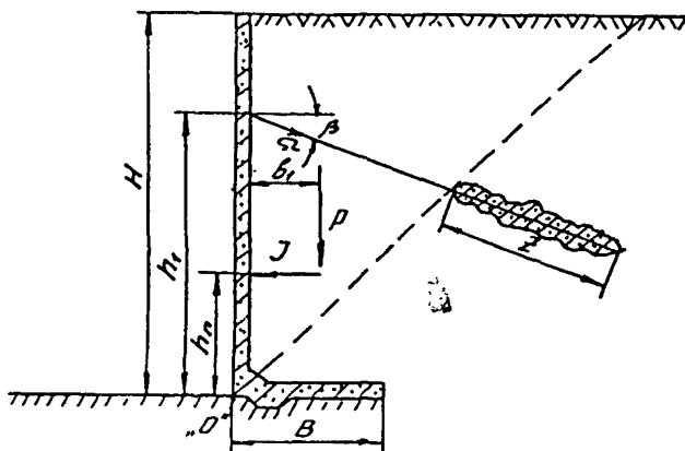
Рис. 35. Схема к расчету сборных заанкеренных подпорных стен
