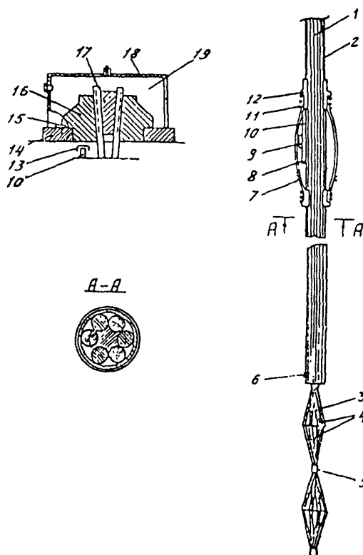
Рис. 21. Грунтовый инъекционный анкер для скальных грунтов.
