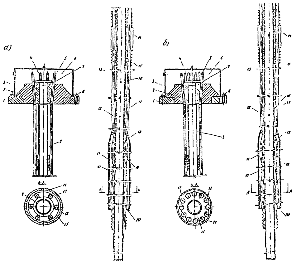
Рис. 19. Грунтовой инъекционный анкер с манжетной трубой при наружном расположении тяг: а - шести; б - двенадцати
