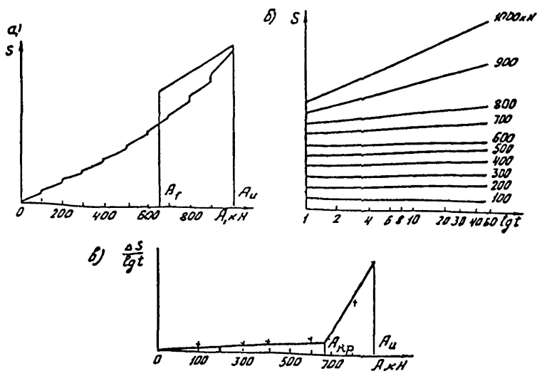
Рис. 30. Графики результатов испытаний: а - S = f(A) ; б - S = f(t) ; в - \frac{\Delta S}{t_{gt}} = f(A)
