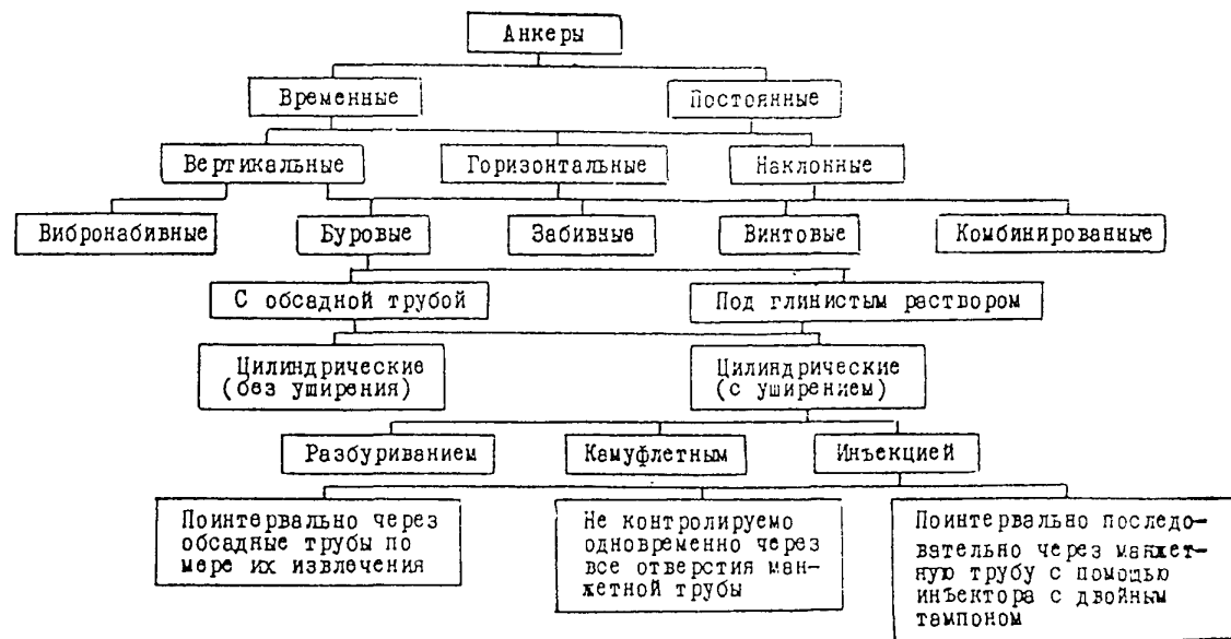
Рис. 2. Классификация анкеров
