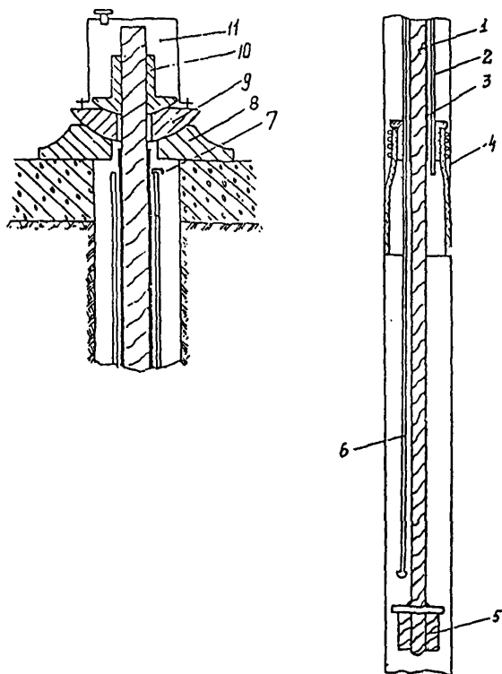
Рис. 15. Временный грунтовый инъекционный анкер с резиновым обтюратором
