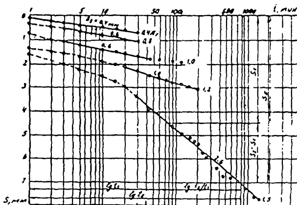
Рис. 27. Графики зависимости деформаций во времени для определения коэффициента ползучести: ---- прямолнейный участок графика, на котором определяется коэффициент ползучести K_s ; - - - криволинейный участок графика
