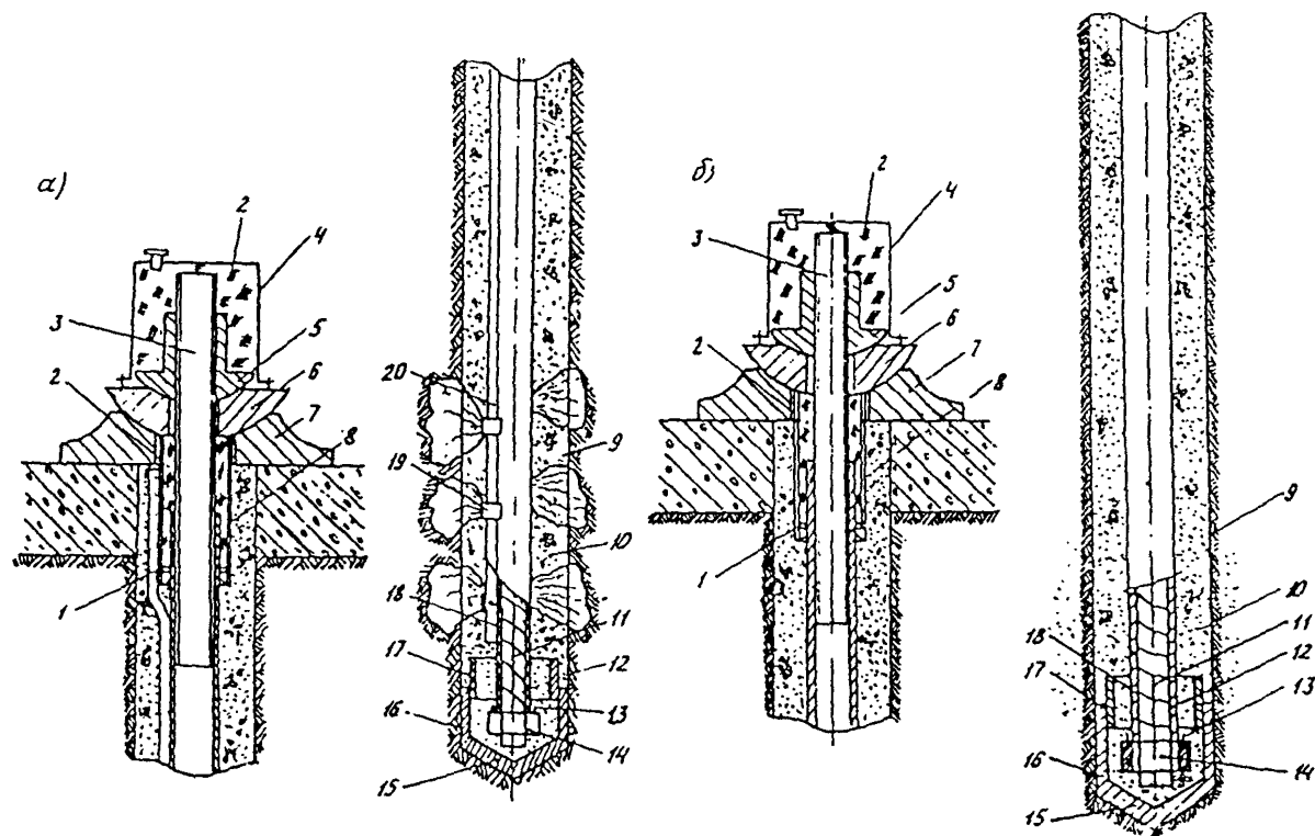
Рис. 22. Грунтовой инъекционный анкер с буровым наконечником для грунтов: а - связных, б - песчаных
