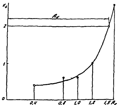
Рис. 28. Пример определения предельной нагрузки
