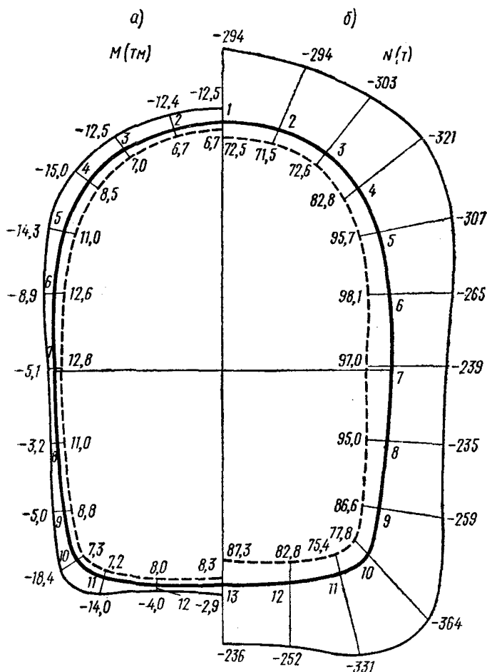
Рис. 2. Расчетные эпюры усилий (изгибающих моментов и продольных сил) для отладочного варианта расчета (значения ординат пунктирной и сплошной линиями см. в тексте)
