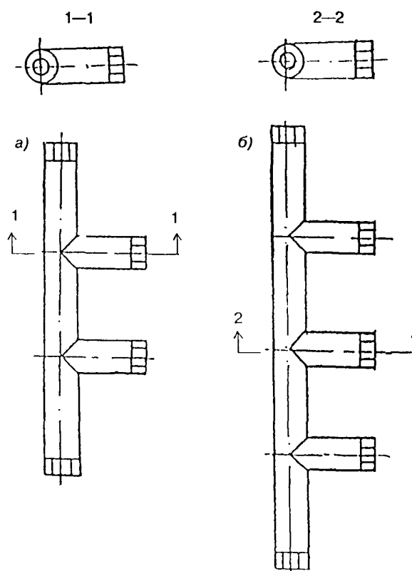
а — с односторонним прямым расположением 2 отводящих штуцеров; б — с односторонним прямым расположением 3 отводящих штуцеров
