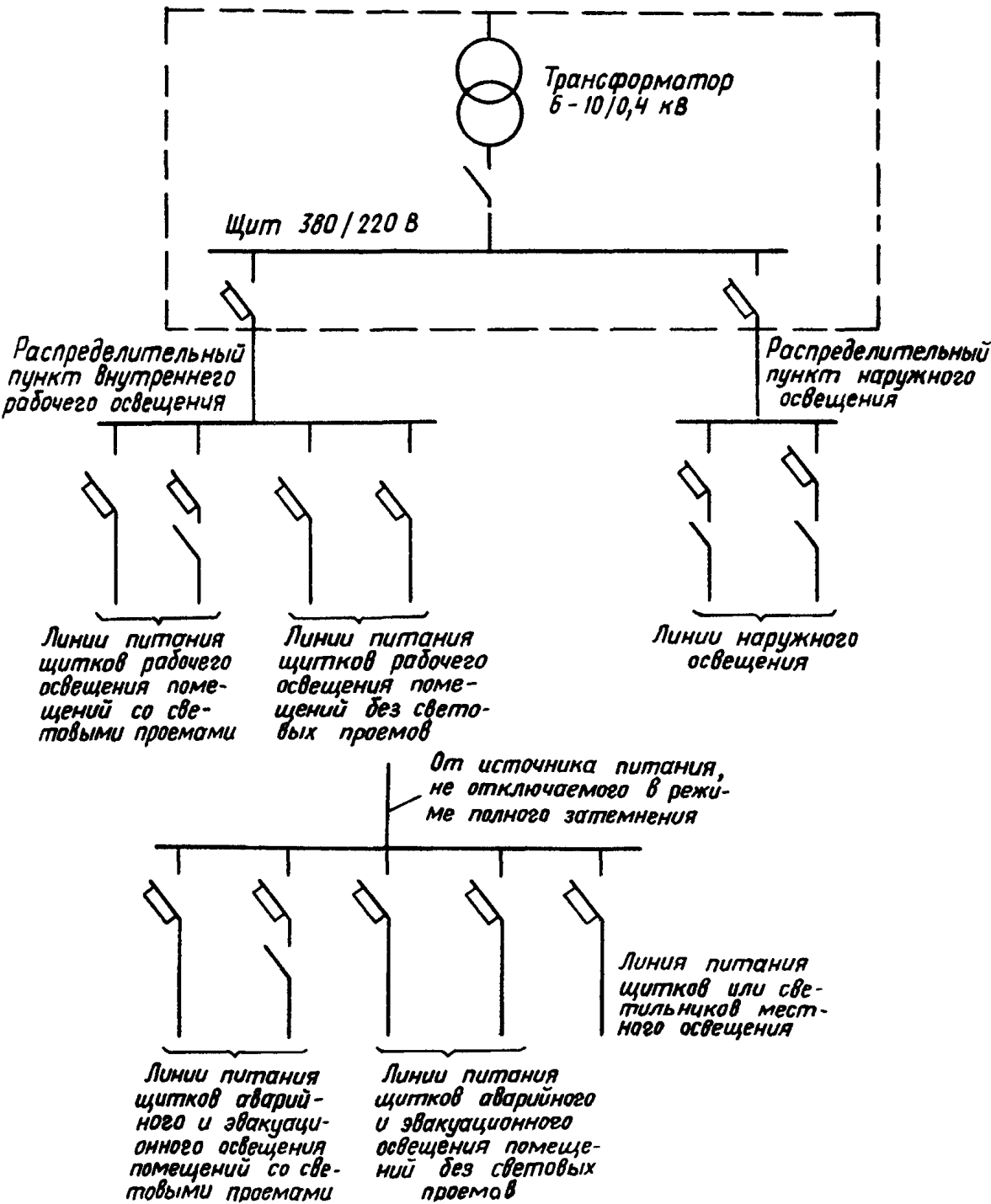
ТИПОВАЯ СХЕМА ЭЛЕКТРОПИТАНИЯ РАБОЧЕГО, АВАРИЙНОГО И ЭВАКУАЦИОННОГО ОСВЕЩЕНИЯ
