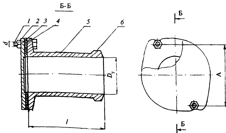
1 — болт; 2 — гайка; 3 — крышка; 4 — прокладка; 5 — корпус; 6 — хвостовик
