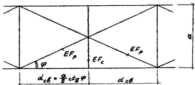
Рис. 5. Треугольные продольные связи
