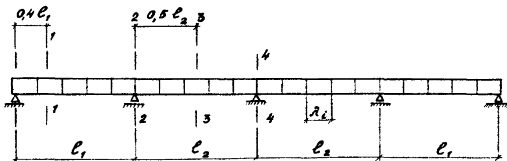
Рис.2. Неразрезные пролетные строения с главными балками ступенчатопеременного сечения трех- и четырех-пролетные
