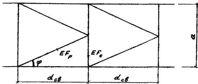
Рис. 4. Полураскосные продольные связи
