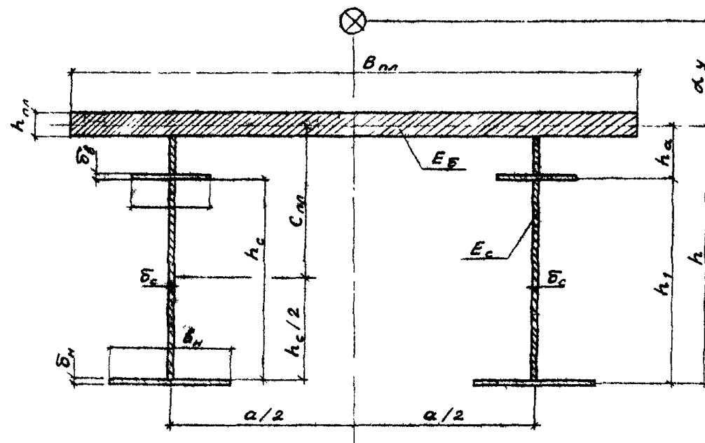
Рис.3. Идеализованное поперечное сечение пролетного строения
