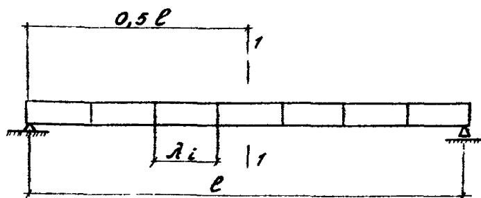
Рис.1. Разрезное пролетное строение с главными балками ступенчатопеременного сечения и расчетным сечением в середине пролета
