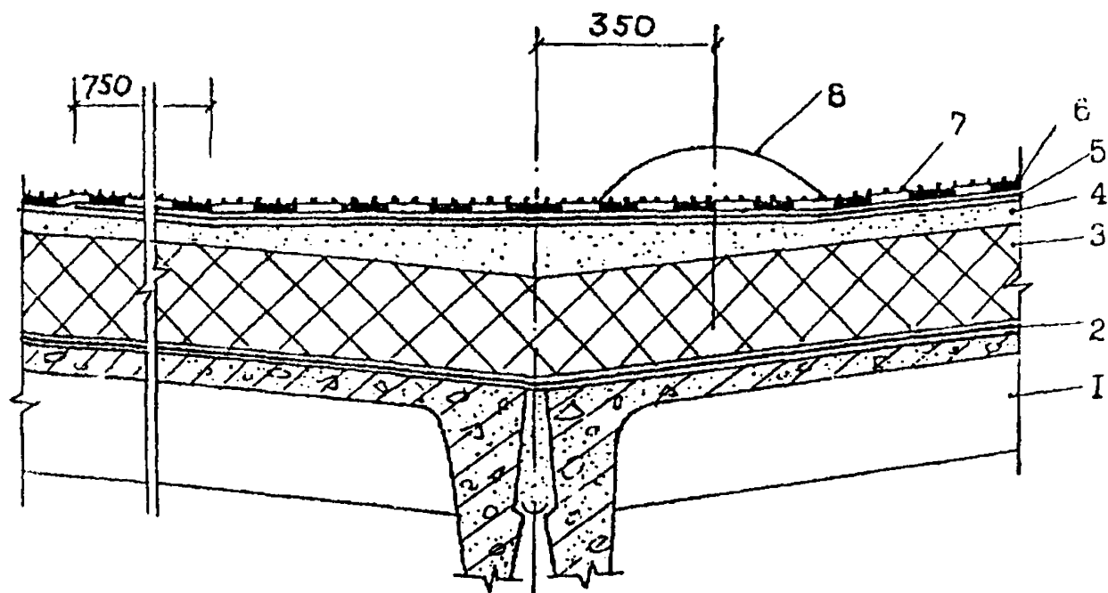
Рис. 8. Ендова кровли
