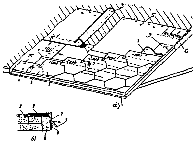
Рис. 20. Конструктивное решение кровли из битумных плиток (шинглас)
