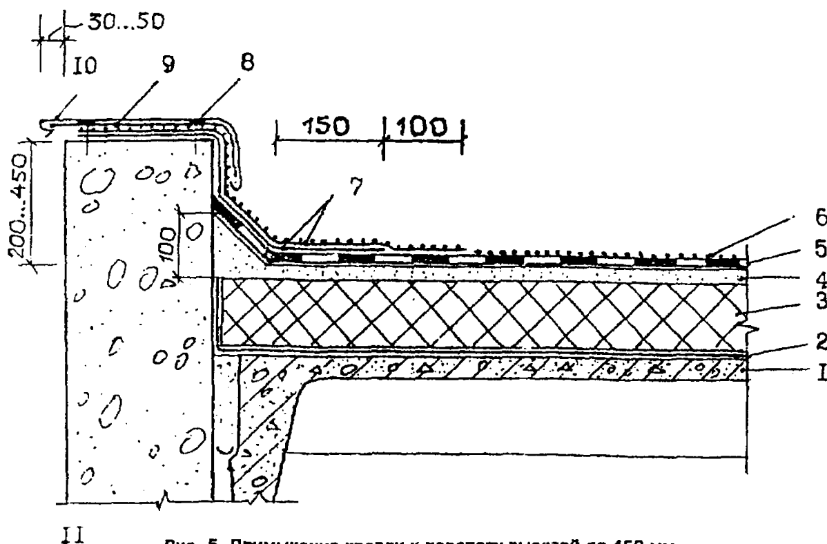
Рис. 5. Примыкание кровли к парапету высотой до 450 мм
