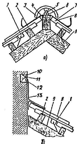
Рис. 21. Узлы черепичной кровли
