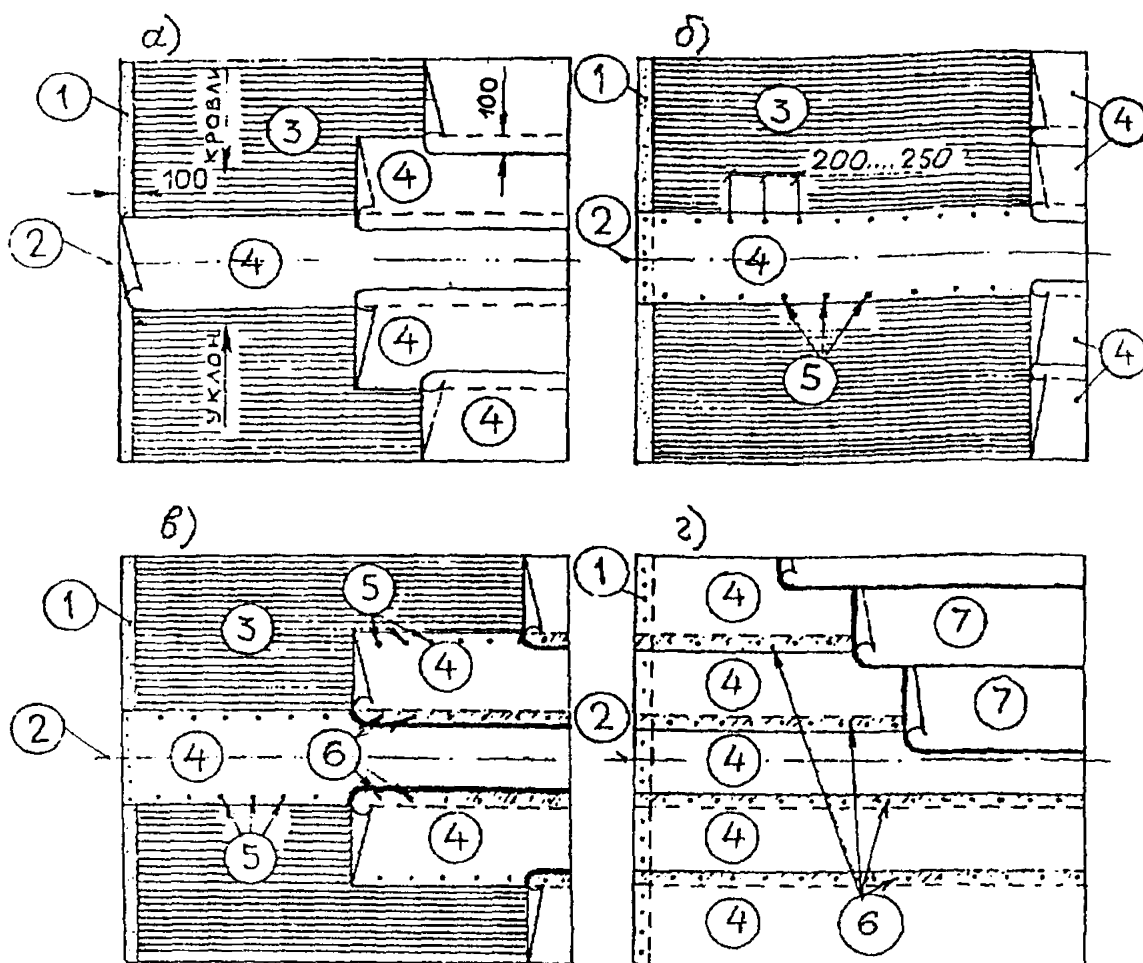
Рис. 9. Пример раскладки рулонных материалов при устройстве водоизоляционного ковра с механическим закреплением нижнего слоя 1 — переходной наклонный бортик (см. рис. 9); 2 — линия водораздела; 3 — основание под кровлю; 4 — нижний слой водоизоляционного ковра; 5 — шайбы с дюбелями; 6 — наклейка полотнищ в местах нахлесток; 7 — верхний (второй) слой водоизоляционного ковра
