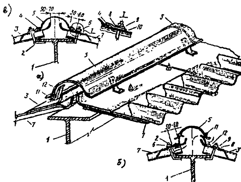
Рис. 18. Устройство коньков
