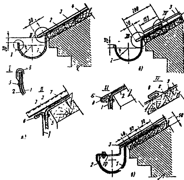
Рис. 25. Устройство подвесного желоба
