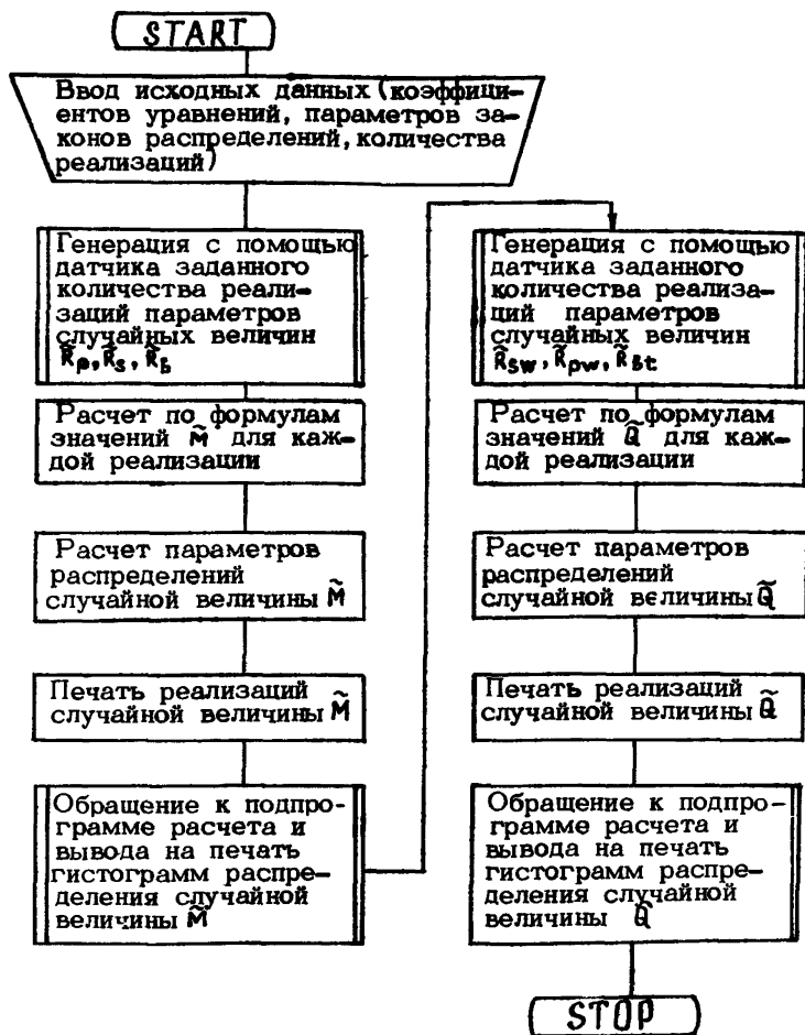
Блок-схема расчета сечений изгибаемых железобетонных элементов на прочность методом статистических испытаний (методом Монте-Карло)
