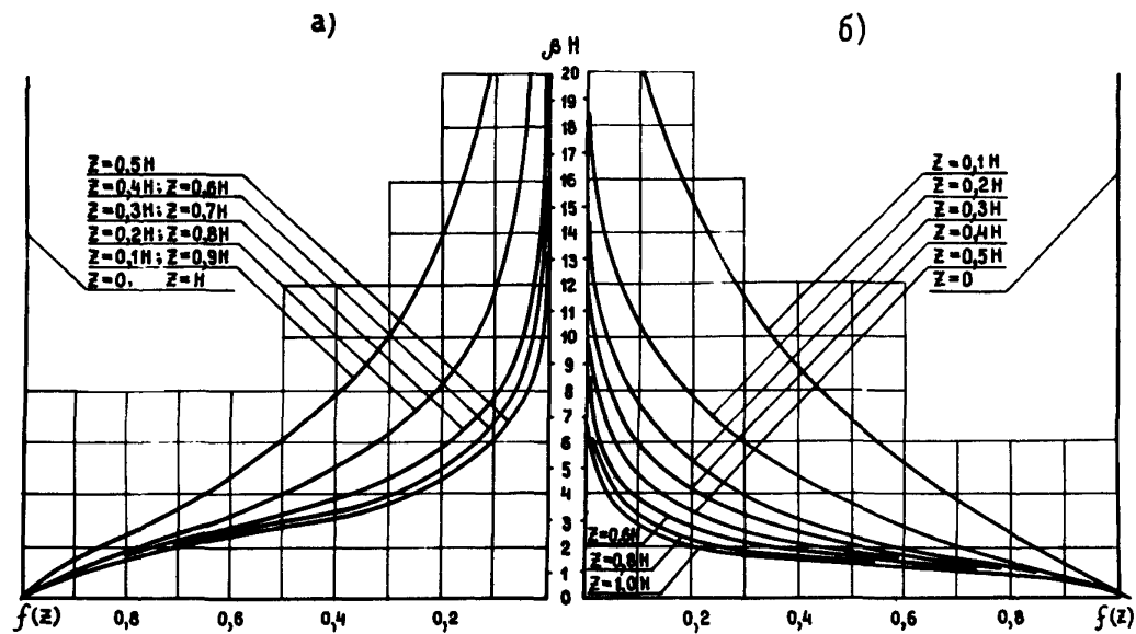
Рис.2. График для определения f(z) при двустороннем (а) и одностороннем (б) отводе воды из дрена
