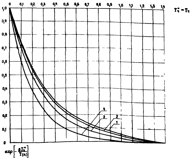
Рис.3. График для определения \exp\left[-\frac{8T_z^*(z)}{F(y)}\right] : 1- d_e=2 м; 2- d_e=1,5 м; 3- d_e=1 м; 4- d_e=0,5 м
