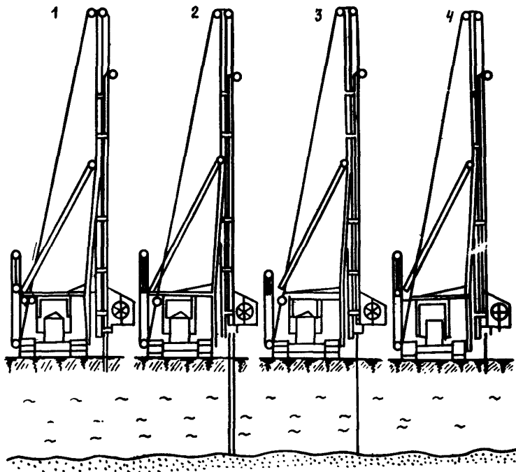
Рис.4. Технология погружения дрен: 1-заправка дрен в обсадную трубу и установка якоря; 2-погружение обсадной трубы с дренаем; 3-извлечение обсадной трубы; 4-начало погружения следующей дрен
