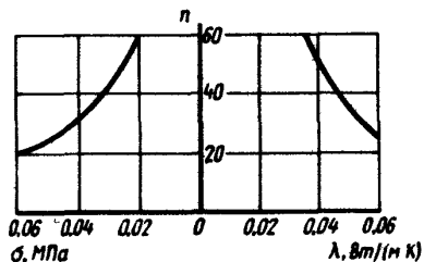
Рис.2. Зависимость прочности \sigma и теплопроводности \lambda пенопласта от его кратности \eta
