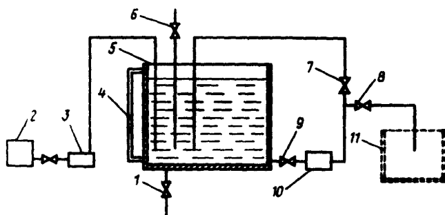
Рис.2. Схема приготовления раствора катализатора: 1,6,7,8,9-вентили; 2-емкость с катализатором; 3-ручной насос; 4-водомерная трубка; 5-бак для раствора катализатора; 10-электронасос; 11-привозная емкость (для раствора катализатора)
