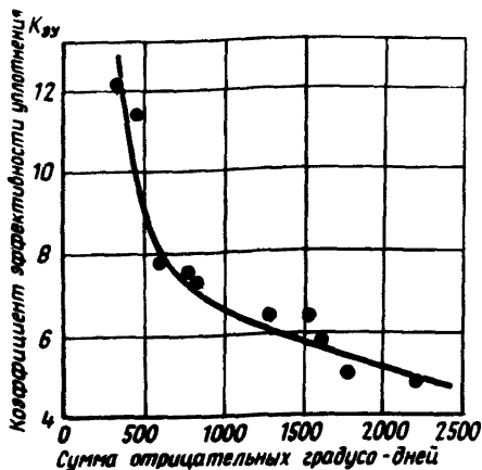
Рис.8. Зависимость коэффициента эффективности утепления грунта K_{3y} БТП от суммы отрицательных градусо-дней
