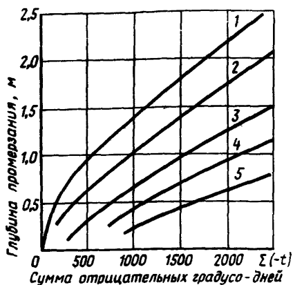
Рис.9. Зависимость глубины промерзания грунта от суммы отрицательных градусо-дней и толщины снегового покрова или пенольда 1-0 м; 2-0,2 м; 3-0,2-0,4 м; 4-0,4-0,6 м; 5- выше 0,6 м
