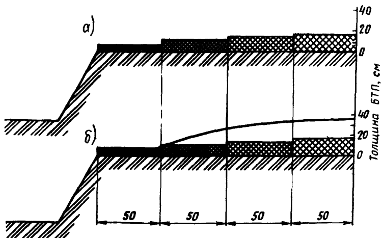
Рис.10. Схема проведения теплоизоляции карьера в Московской обл. ( H_{пр}=140 см): а-утепление БТП и снегом (пенольдом) при их средней толщине 20 см; б-утепление только БТП
