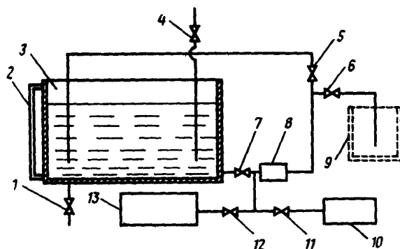
Рис.1. Схема приготовления раствора смолы и пенообразователя: 1,4,5,6,7,11,12- вентили; 2-водомерная трубка; 3-бак для раствора; 8-электронасос; 9-привозная емкость для раствора; 10-емкость с пенообразователем; 13-емкость со смолой
