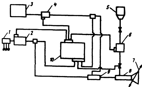
Рис.6. Принципиальная схема установки ПМП-2 конструкции СевНИИГиМа: 1 - электромотор; 2 - компрессор; 3 - емкость с раствором смолы и пенообразователя; 4, 6 - насосы; 5 - емкость с раствором катализатора; 7 - устройство для механического распределения пены; 8, 9 - камеры пеногенератора; 10 - пульт управления
