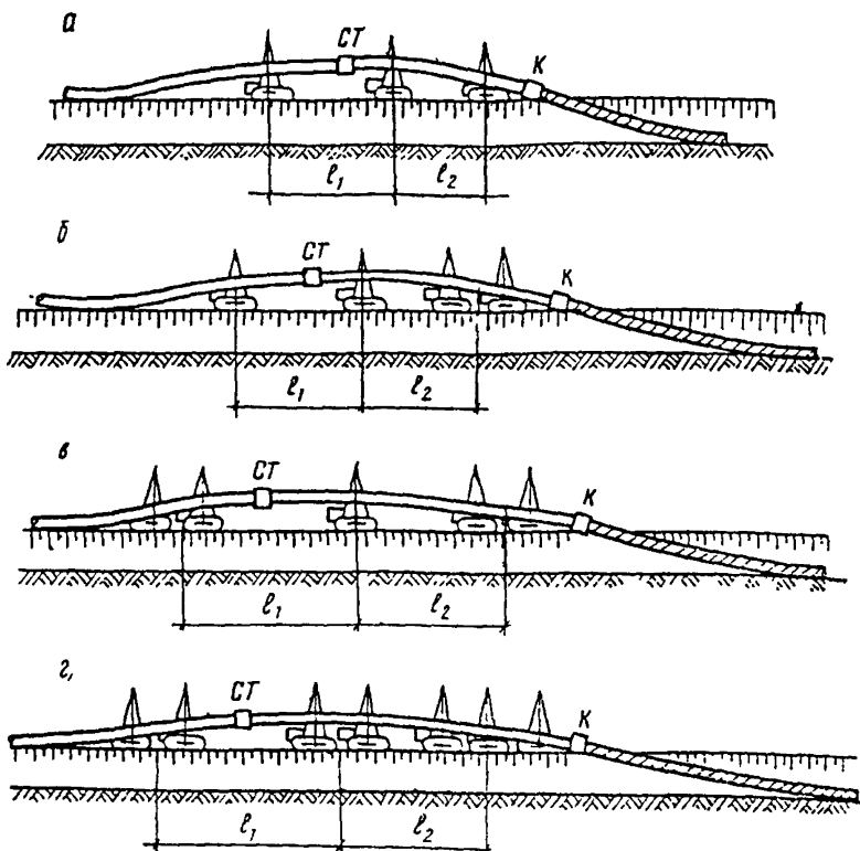
Рис.10. Схемы расстановки трубоукладчиков и машин в изоляционно-укладочной колонне при совмещенном способе производства работ для трубопроводов различных диаметров:
