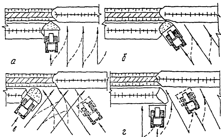
Рис.7. Схемы производства работ по засыпке уложенного трубопровода бульдозером: а-прямолинейными проходами; б-косоперечными параллельными проходами; в-косоперекрестными проходами; г-комбинированным способом
