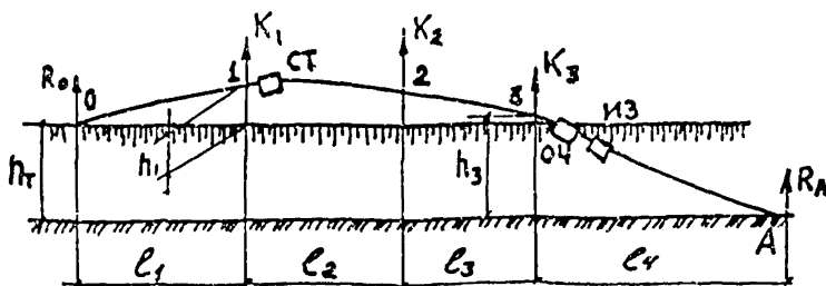
Расчетно-технологическая схема
