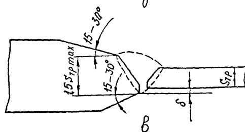
Рис.2. Варианты сборки стыков разнотолщинных элементов: а - совпадение наружных диаметров трубы и детали; б - совпадение внутренних диаметров; в - сборка разнотолщинных элементов при несовпадении диаметров; S - номинальная толщина стенки детали; S_{гр} - нормативная толщина стенки трубы; \delta - смещение кромок при сборке стыка; D_{гр} - наружный нормативный диаметр трубы; D_{сб} - сборочный диаметр D_{сб} = (D_{гр} - 2S_{гр}) \pm 1 мм
