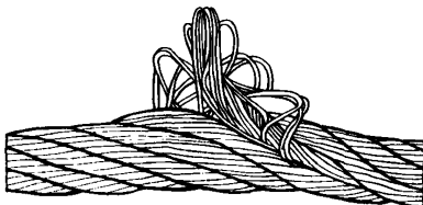
Рис. 10. Выдавливание сердечника
