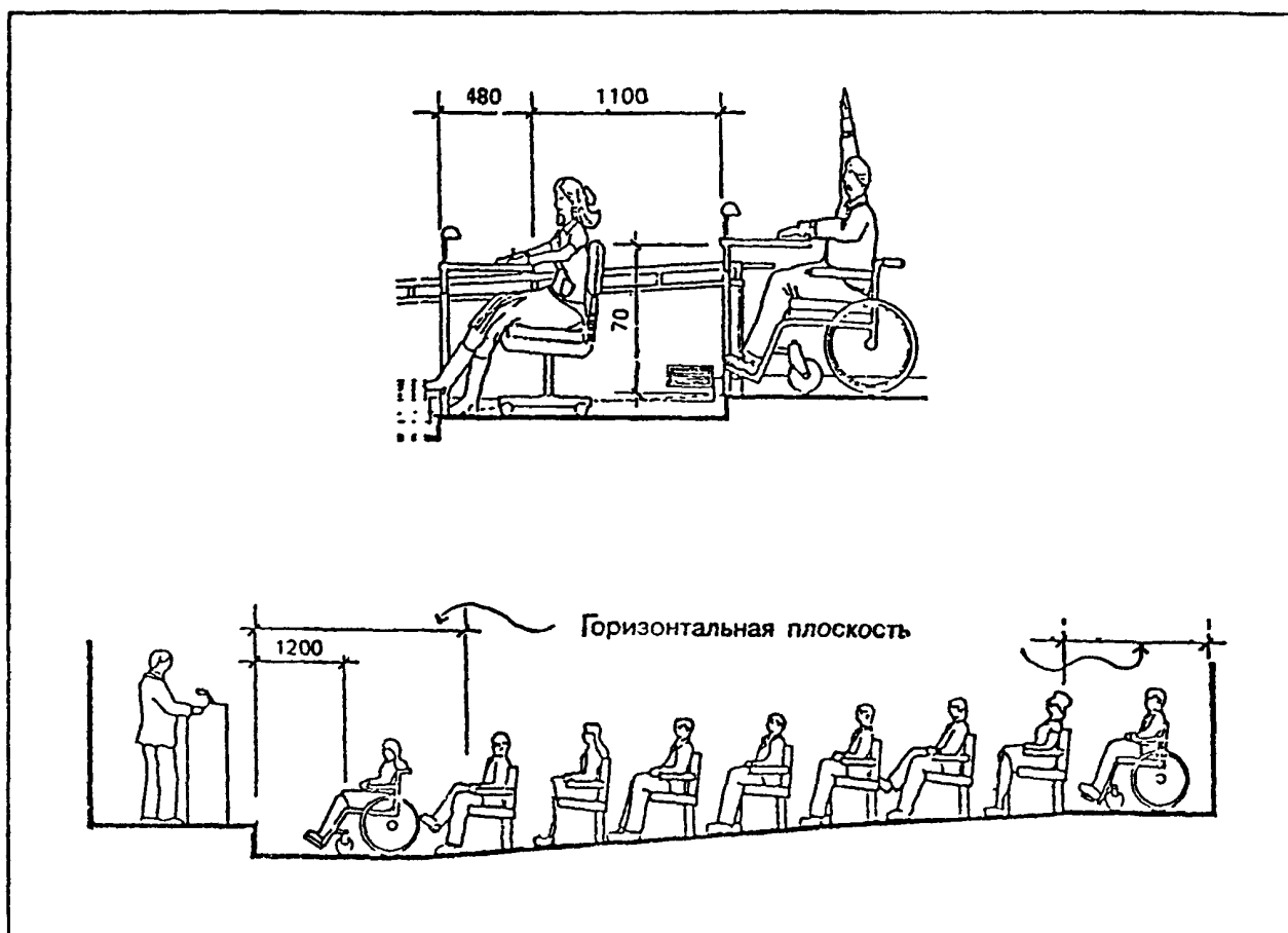
Размещение оборудования и места для инвалидов-колясочников в лекционных залах
