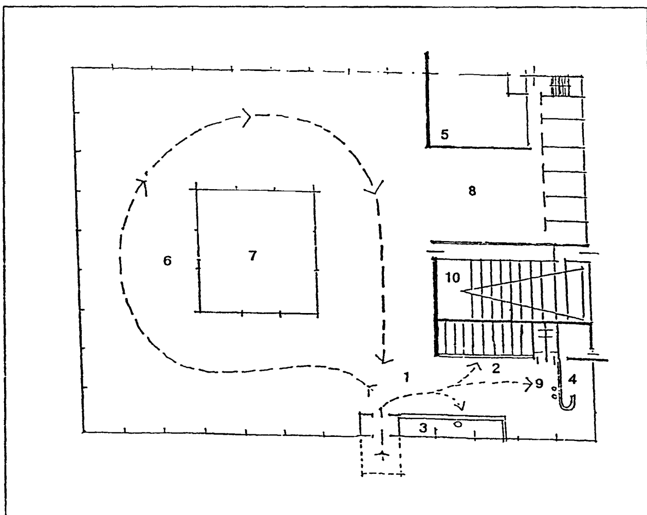
Зонирование основных помещений музея при одноэтажной композиции здания музея, посещаемого инвалидами
