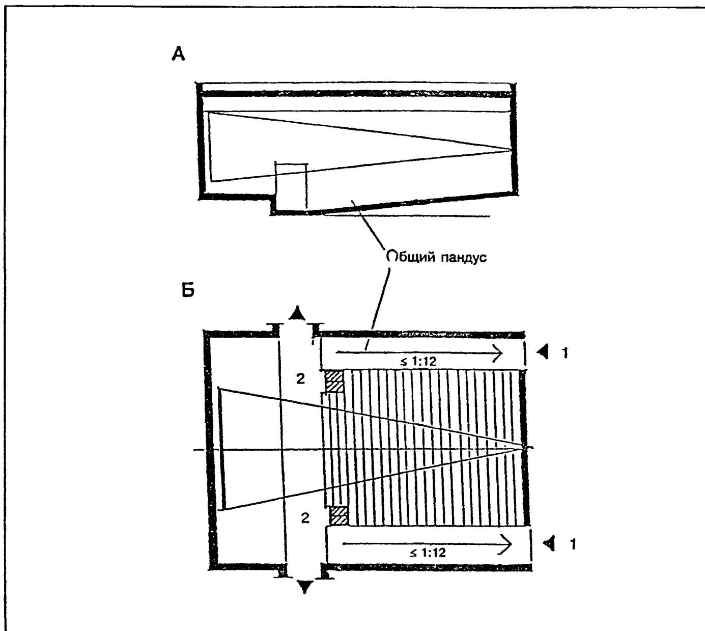
Пример решения загрузки и эвакуации инвалидов-колясочников в кинозалах с уклоном пандусов менее 1:12 А — разрез; Б — план; 1 — пути загрузки и эвакуации; 2 — места для инвалидов
