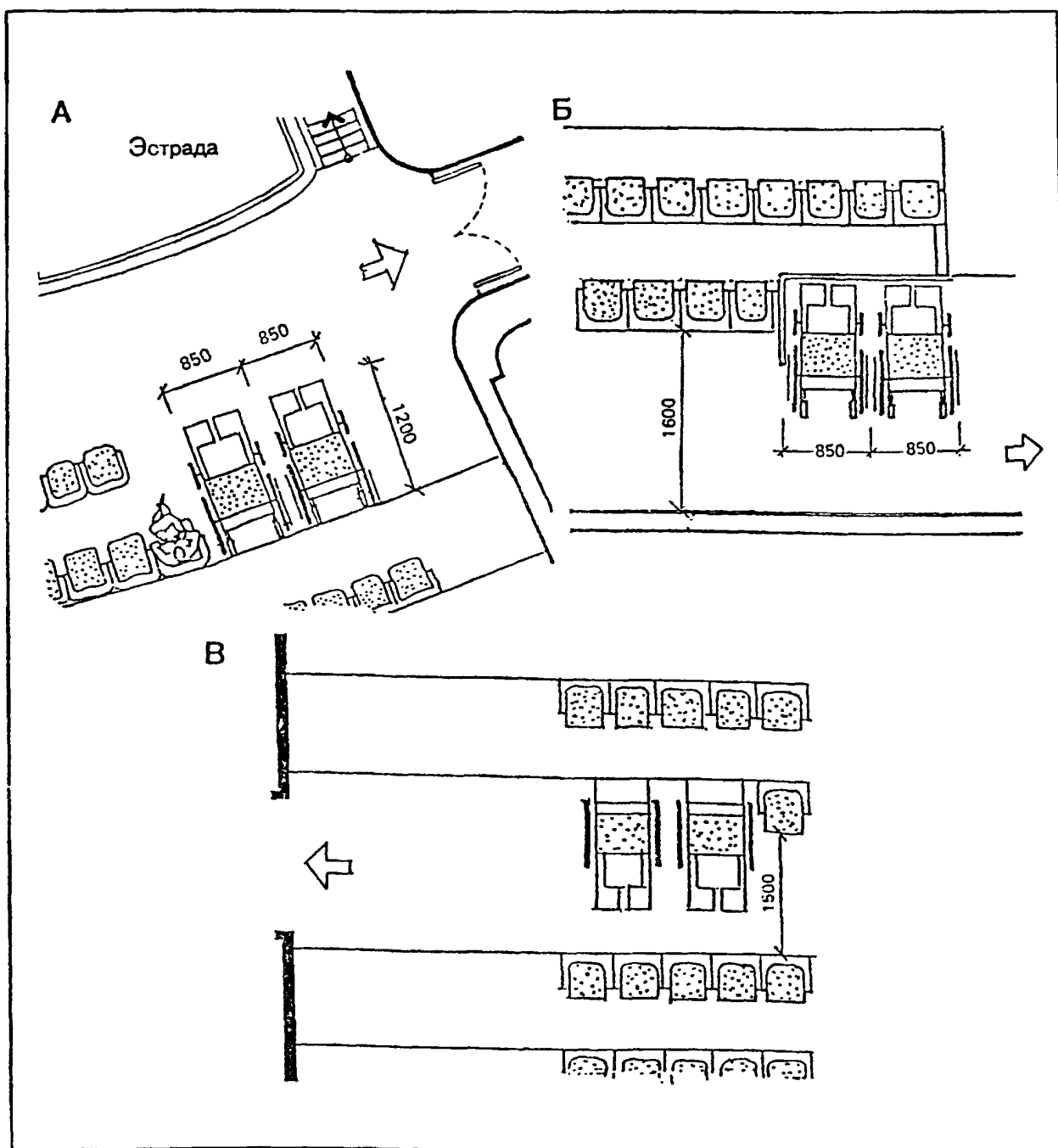
Оборудование мест для инвалидов-колясочников в зрительных залах А — в первом ряду; Б — в последнем ряду; В — в поперечном проходе
