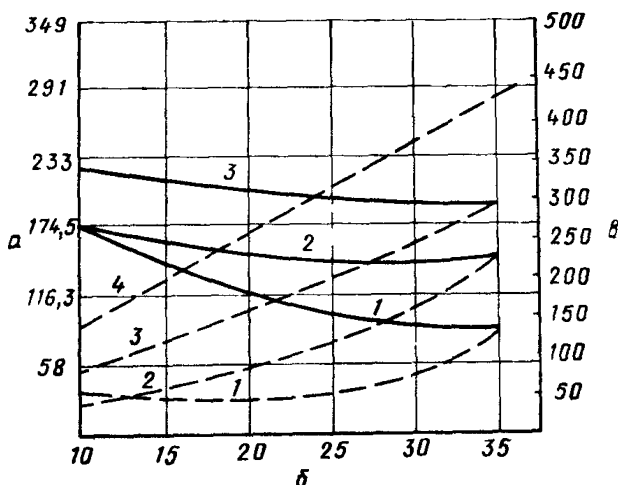
Рис. 3. Зависимость количества тепла и влаги, выделяемых человеком, от температуры воздуха в помещении и характера работы a – тепловыделение, Вт; b – температура воздуха, ^{\circ}\text{C} ; v – влаговыделение, г/ч — — — полное количество тепла, — — — — тепло, идущее на испарение влаги; 1 – человек в покое; 2 – легкая работа в учреждении; 3 – физическая работа; 4 – тяжелая физическая работа
