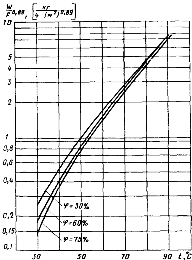
Рис. 4. Влаговыведения с открытой водной поверхностью технологического оборудования в зависимости от относительной влажности внутреннего воздуха \varphi , % и температуры воды t , °C, для t_{\text{в}} = 16^\circ\text{C} , P_{\text{д}} = 1,01 \cdot 10^5 Па
