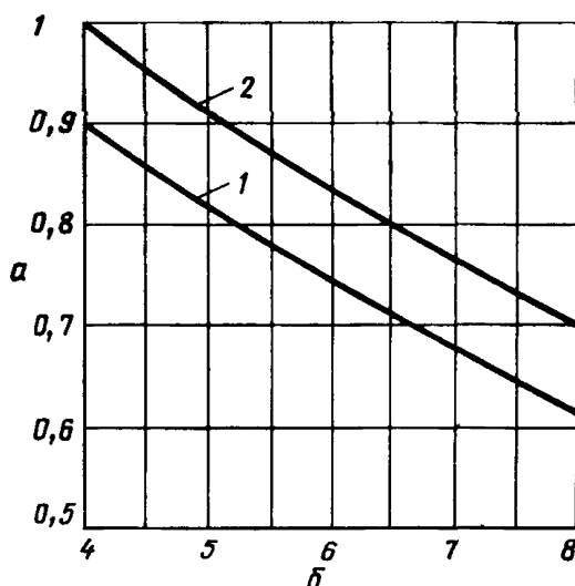
Рис. 2 Средние значения температурного градиента \Delta , ^{\circ}\text{C}/\text{м} , в зависимости от высоты помещения и теплонапряженности q , \text{Вт}/\text{м}^2 a – температурный градиент \Delta , ^{\circ}\text{C}/\text{м} ; h – высота помещения, м; 1 – до 23 \text{Вт}/\text{м}^2 ; 2 – до 46 \text{Вт}/\text{м}^2
