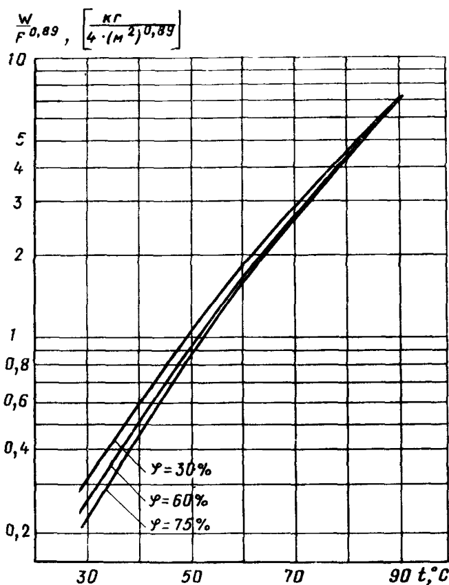
Рис. 5. Влаговыделения с открытой водной поверхности технологического оборудования в зависимости от относительной влажности внутреннего воздуха \varphi , %, и температура воды t , °C, для t_{\text{в}} = 22^\circ\text{C} и P_{\delta} = 1,01 \cdot 10^5 Па
