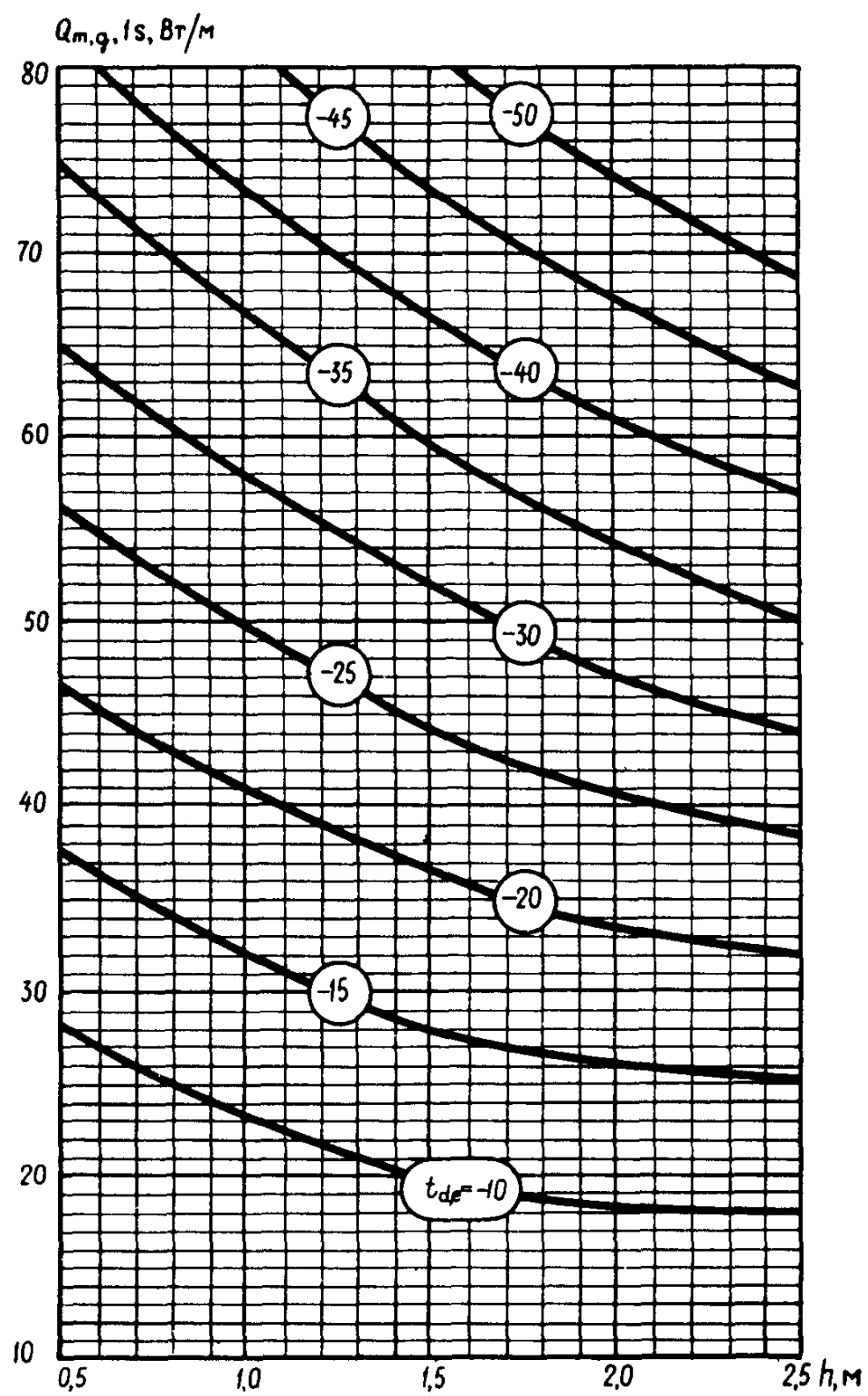
Черт. 3. Графики зависимости Q_{m,g,1s} от h и t_{d,e}
